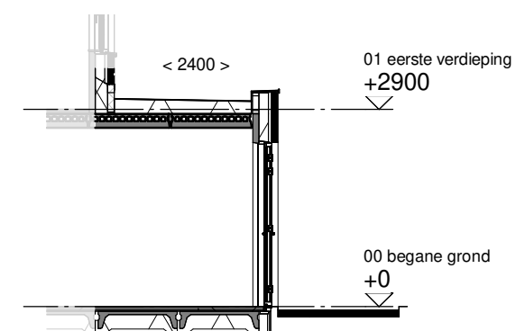
Doorsnede schaal 1:100
