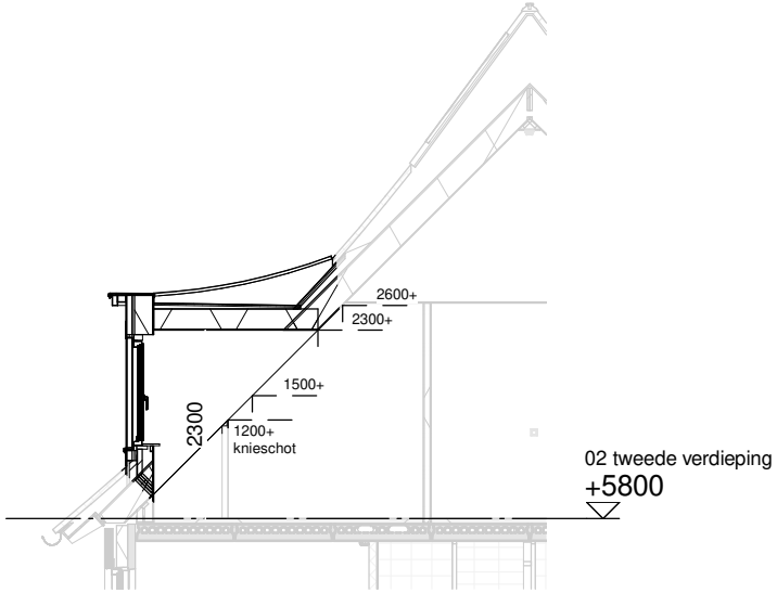
Doorsnede schaal 1:100
