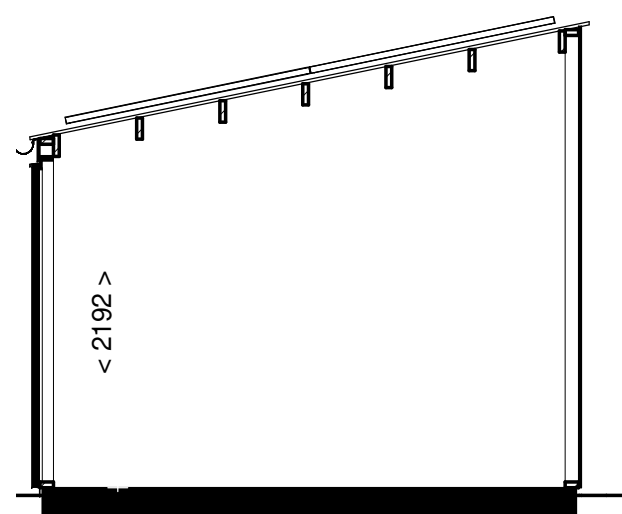
Doorsnede B-B
