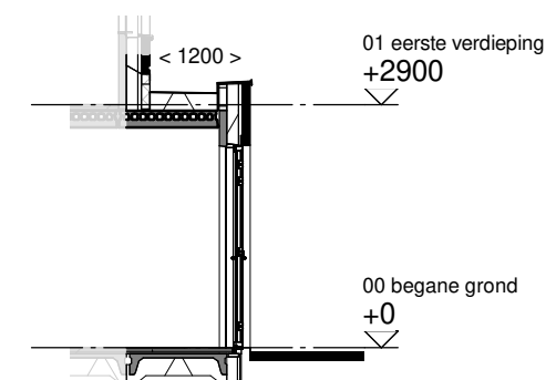
Doorsnede schaal 1:100
