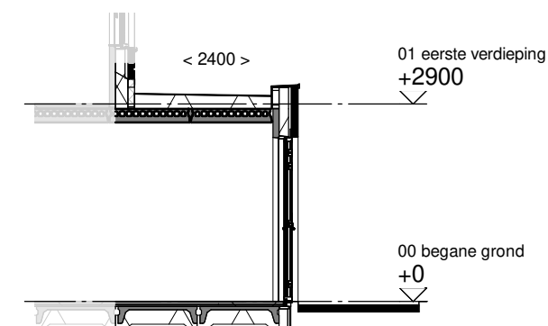
Doorsnede schaal 1:100
