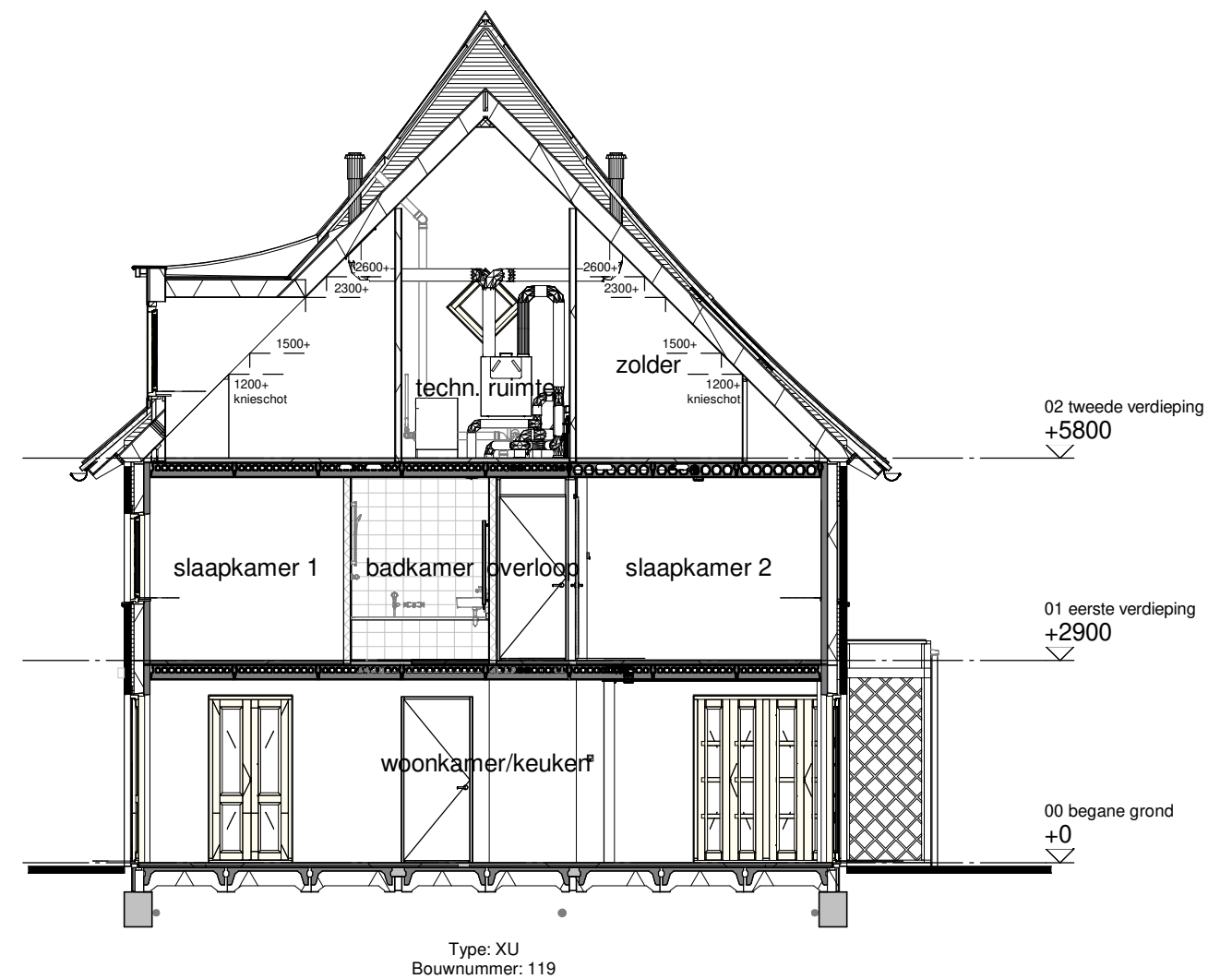
Doorsnede B
