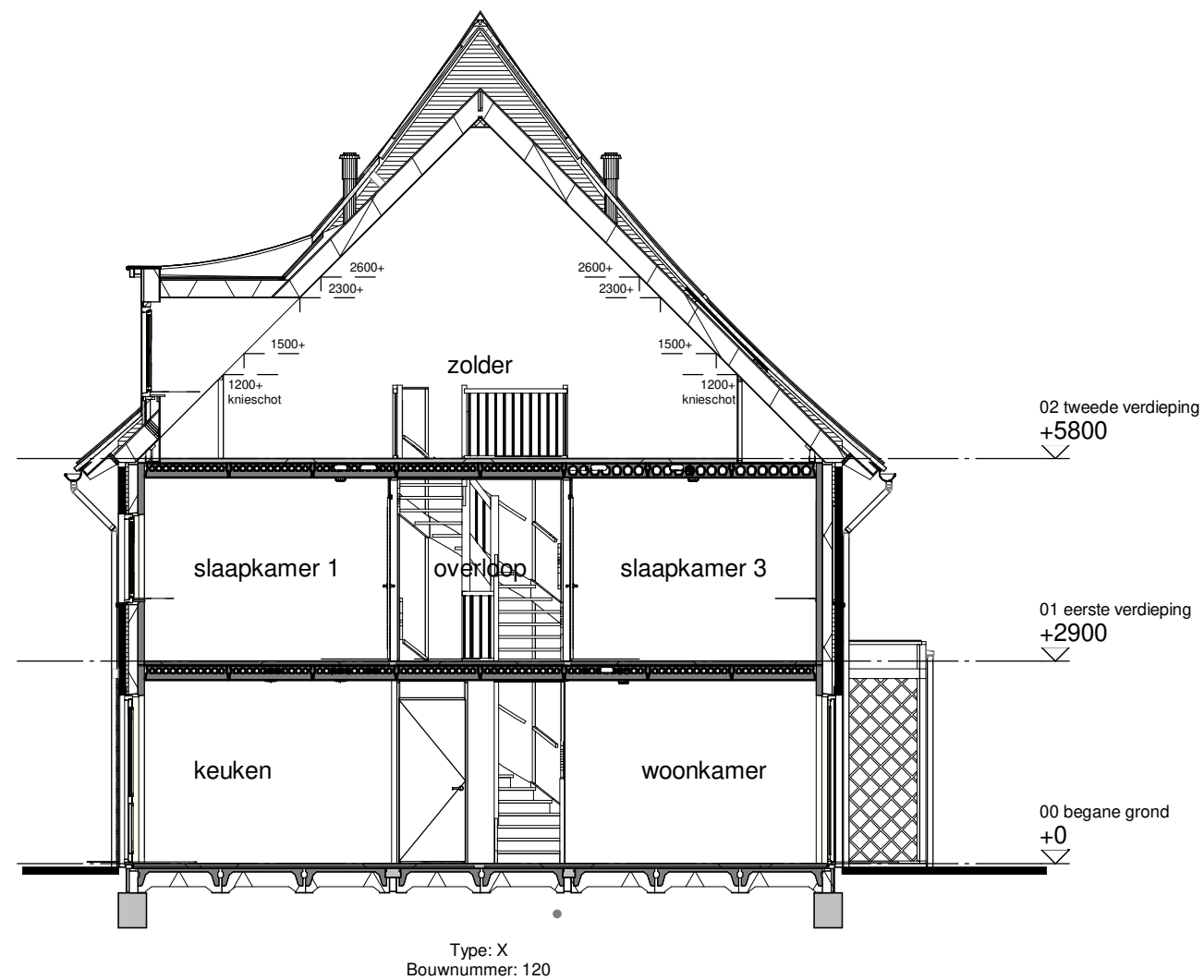
Doorsnede A
