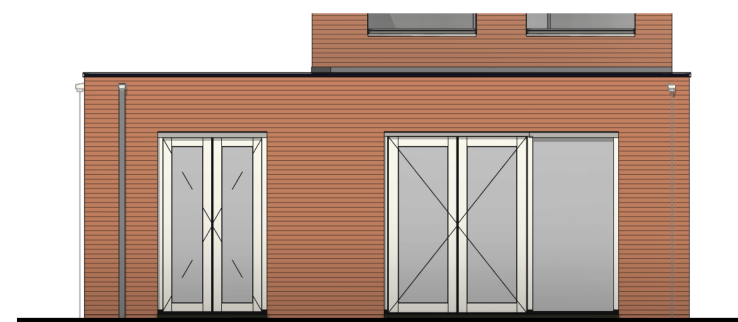
Achtergevel schaal 1:100
