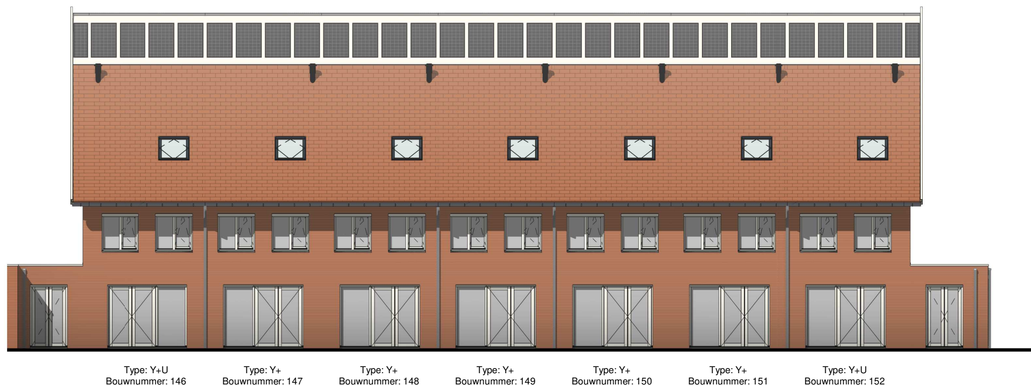
Achtergevel
