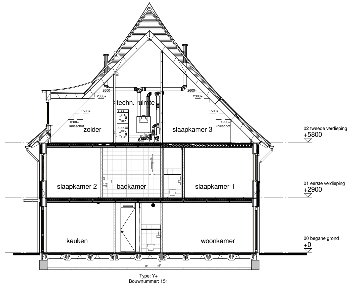
Doorsnede B
