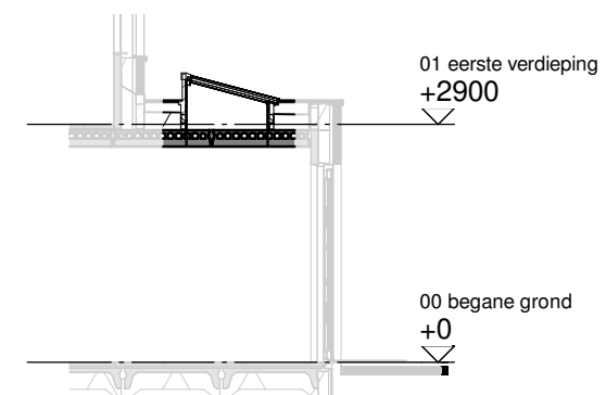
Doorsnede schaal 1:100
