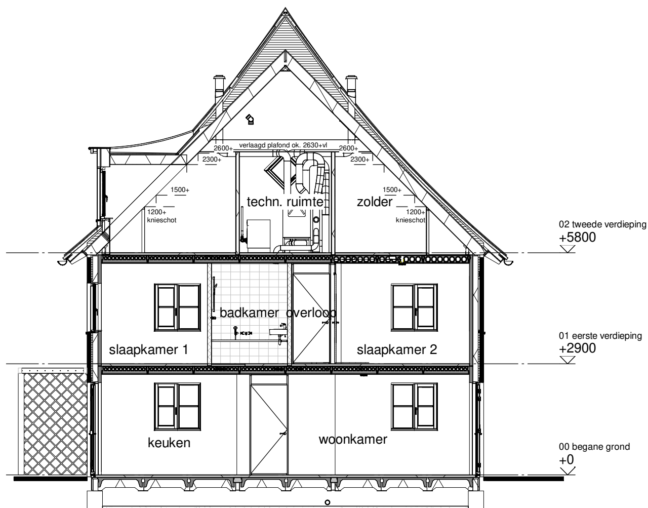
Doorsnede A
