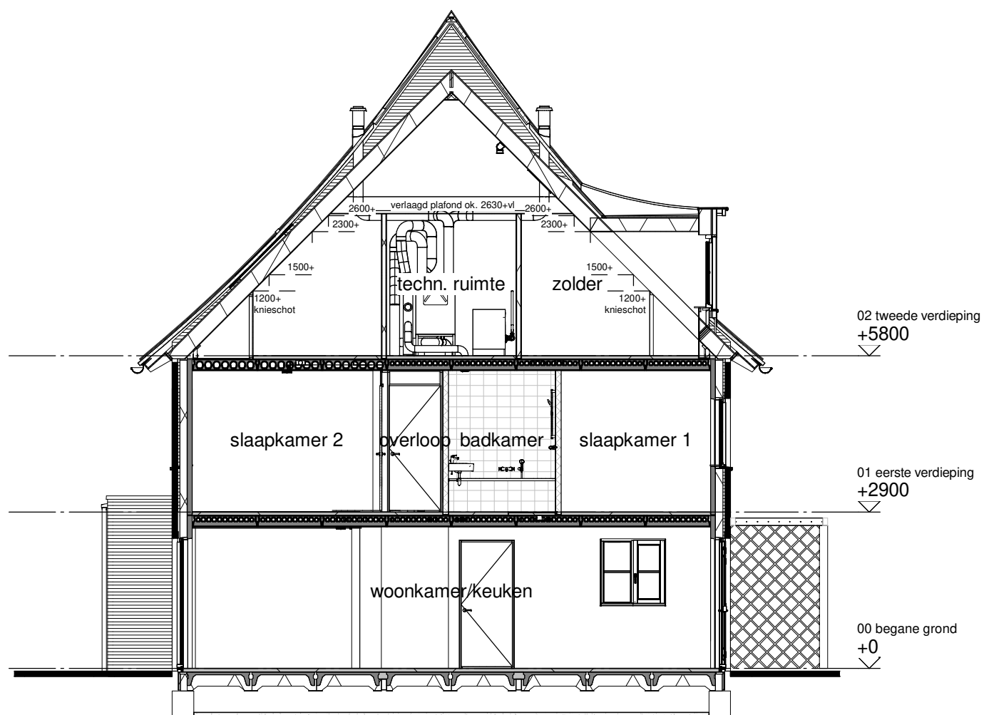
Doorsnede B
