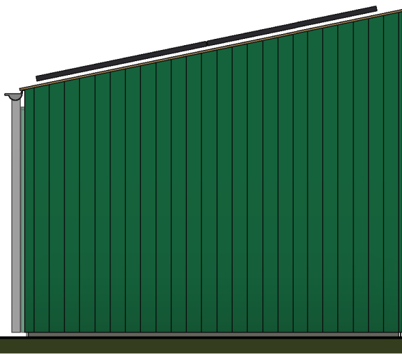
Rechter zijgevel
