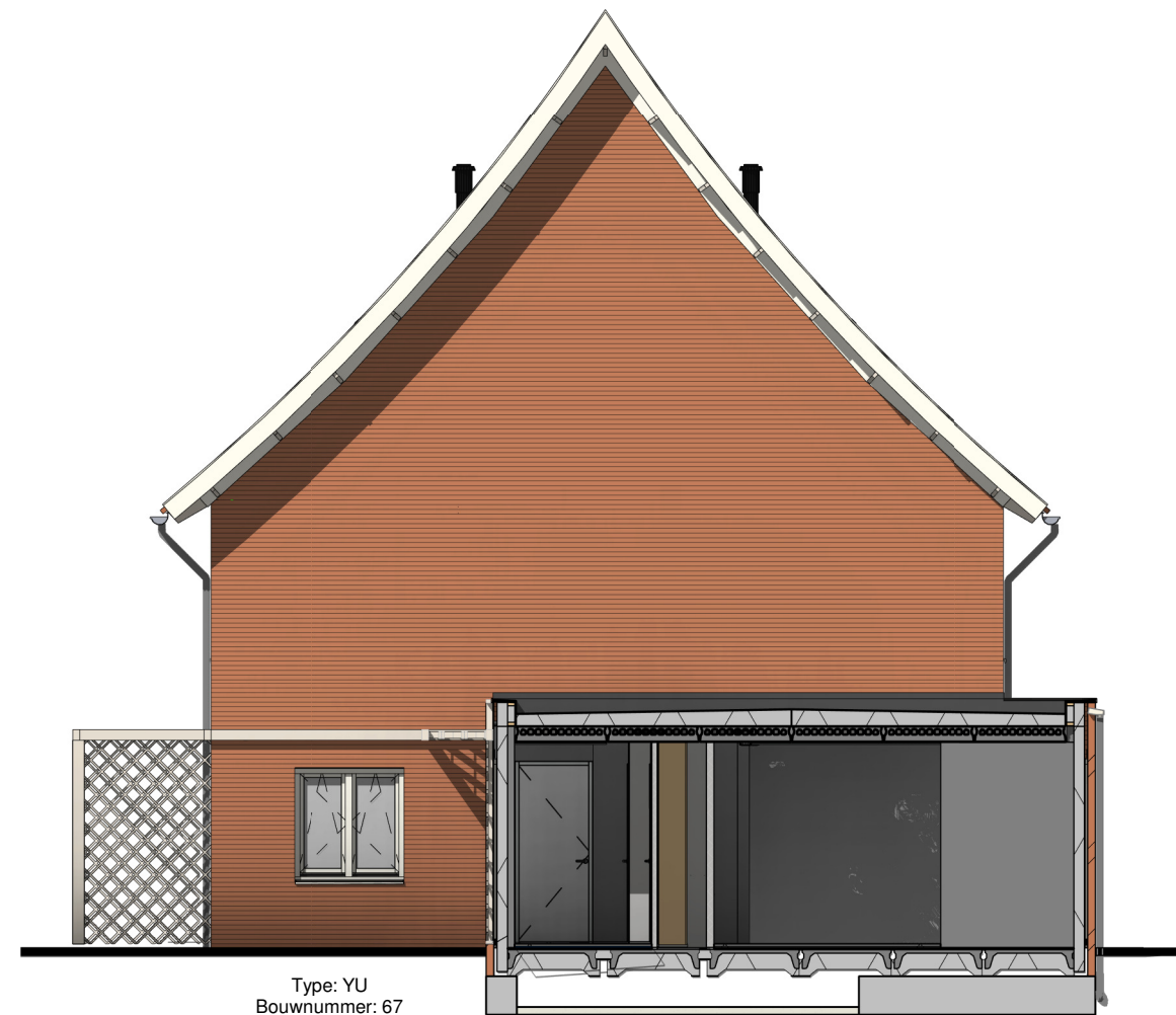
Rechter zijgevel
