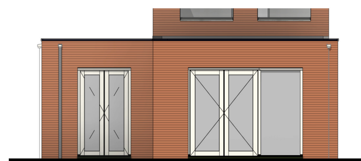
Achtergevel schaal 1:100
