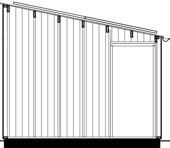
Doorsnede B-B
