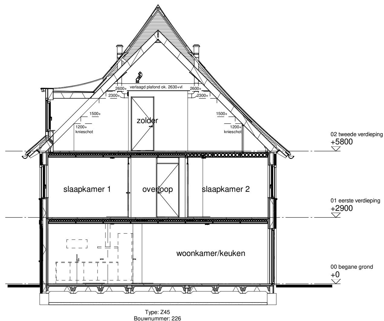
Doorsnede A
