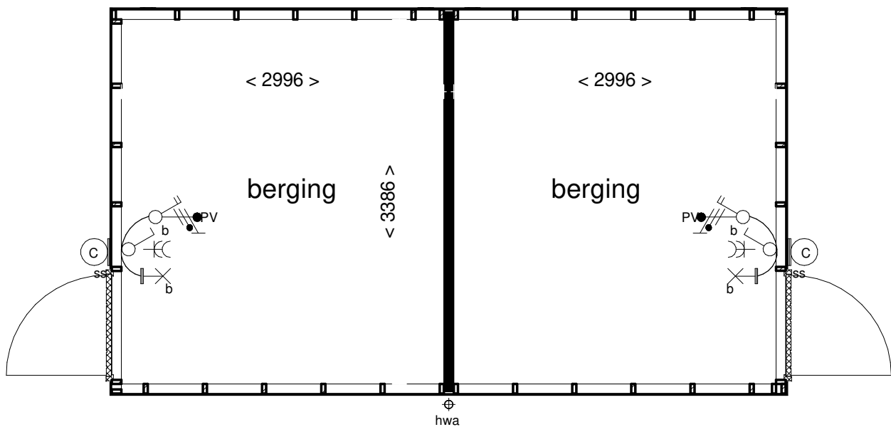
Begane grond
