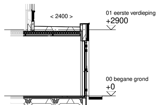
Doorsnede schaal 1:100
