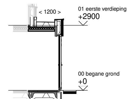
Doorsnede schaal 1:100
