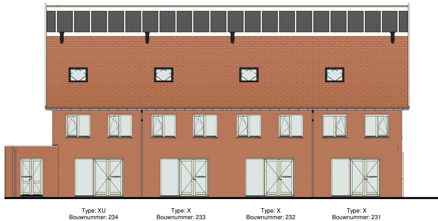
Achtergevel
