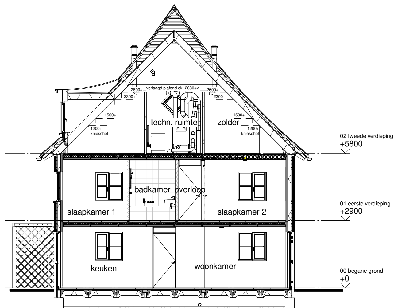
Doorsnede A
