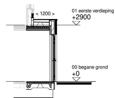
Doorsnede schaal 1:100
