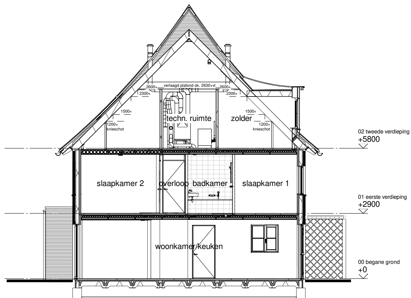
Doorsnede B
