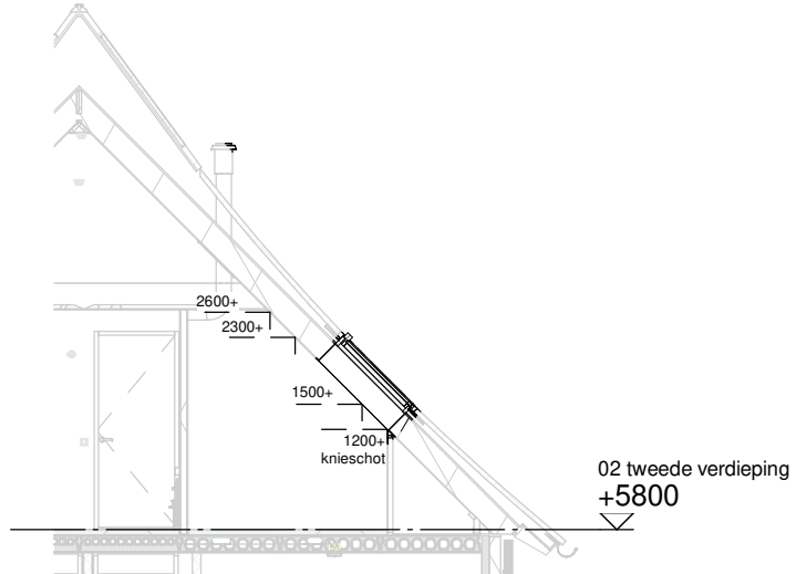
Doorsnede schaal 1:100
