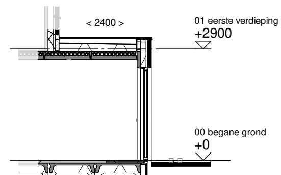
Doorsnede schaal 1:100
