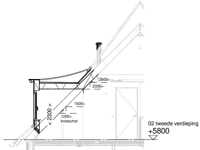
Doorsnede schaal 1:100
