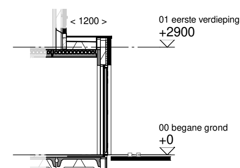
Doorsnede schaal 1:100
