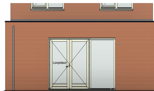
Achtergevel schaal 1:100
