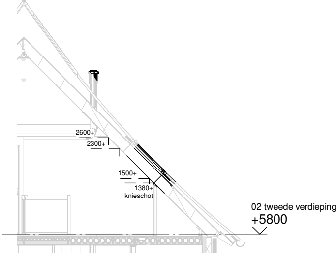
Doorsnede schaal 1:100
