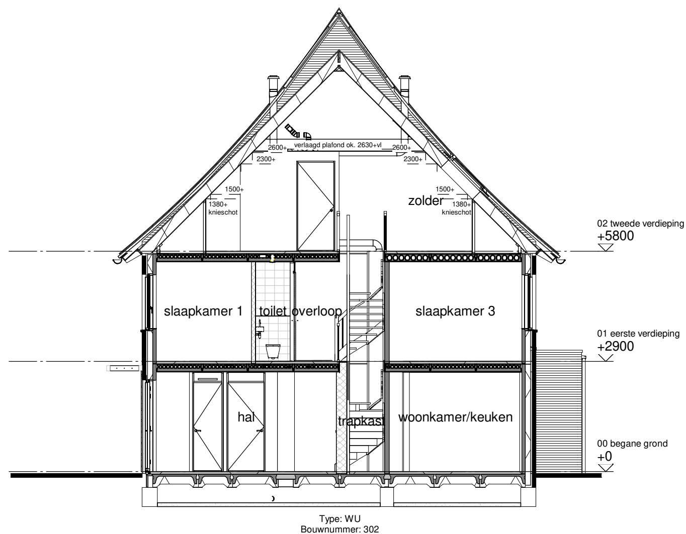
Doorsnede A
