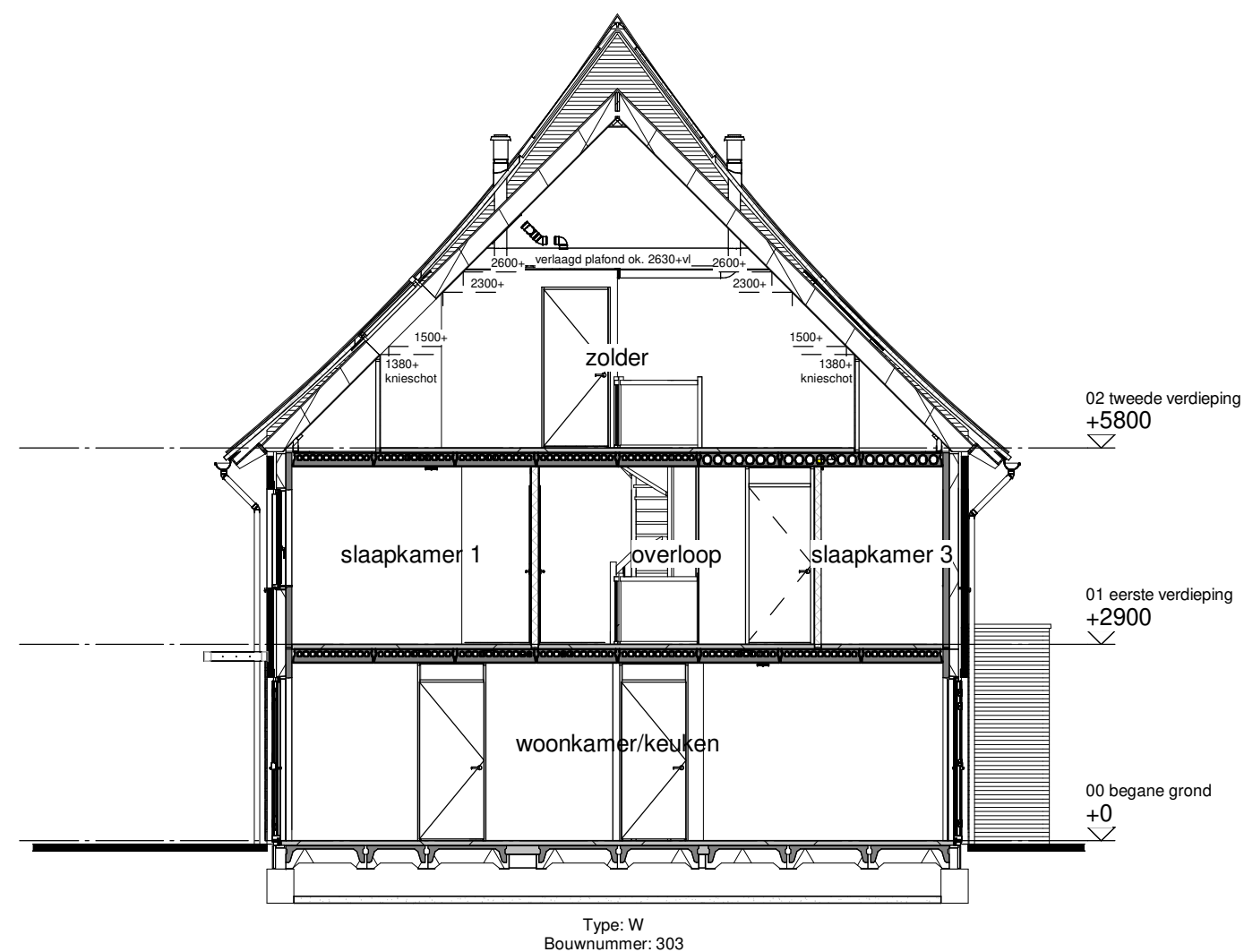
Doorsnede B
