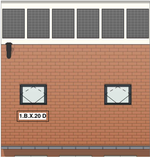
Voorgevel schaal 1:100
