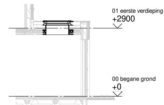
Doorsnede schaal 1:100
