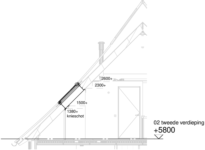
Doorsnede schaal 1:100
