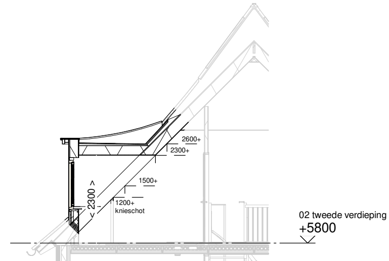
Doorsnede schaal 1:100
