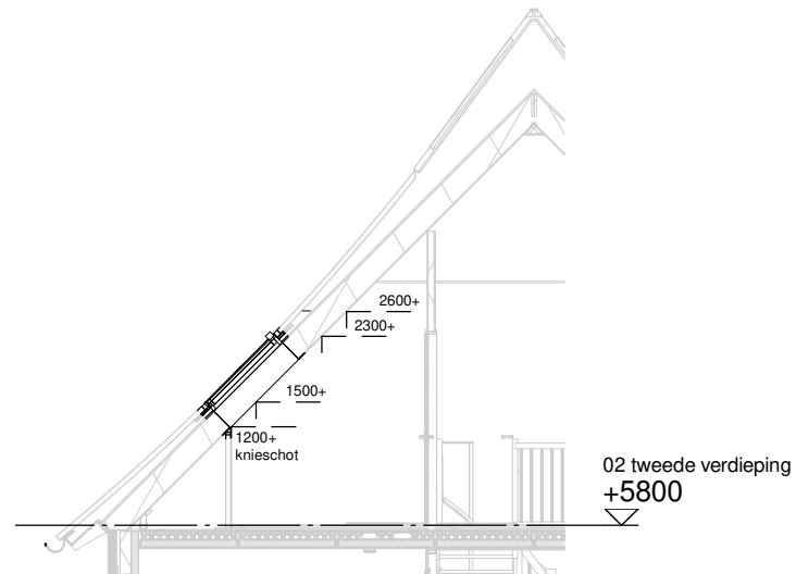
Doorsnede schaal 1:100
