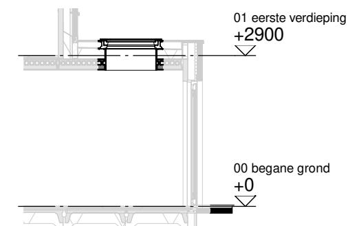
Doorsnede schaal 1:100
