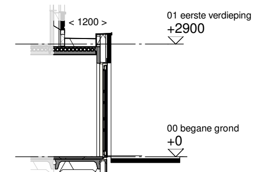
Doorsnede schaal 1:100
