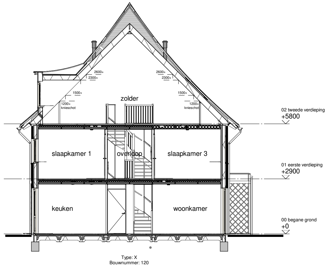
Doorsnede A
