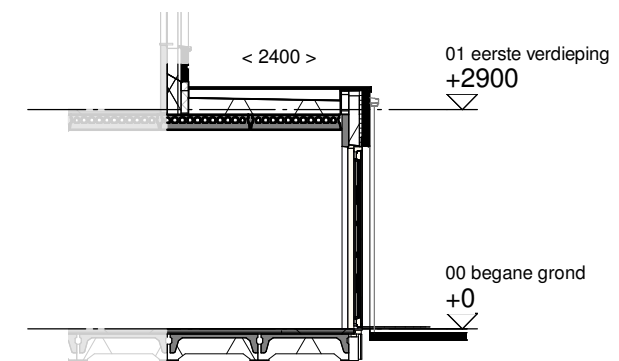
Doorsnede schaal 1:100
