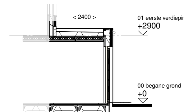
Doorsnede schaal 1:100
