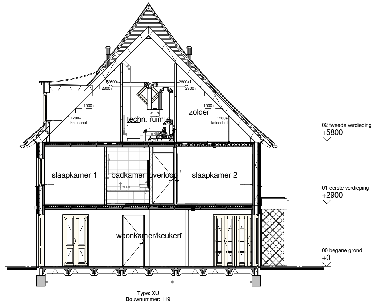
Doorsnede B
