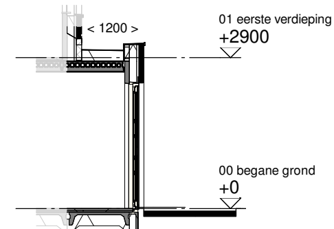
Doorsnede schaal 1:100
