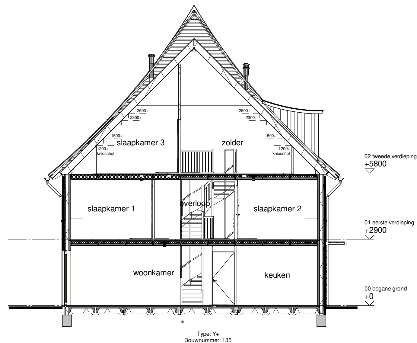
Doorsnede B
