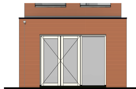
Achtergevel schaal 1:100
