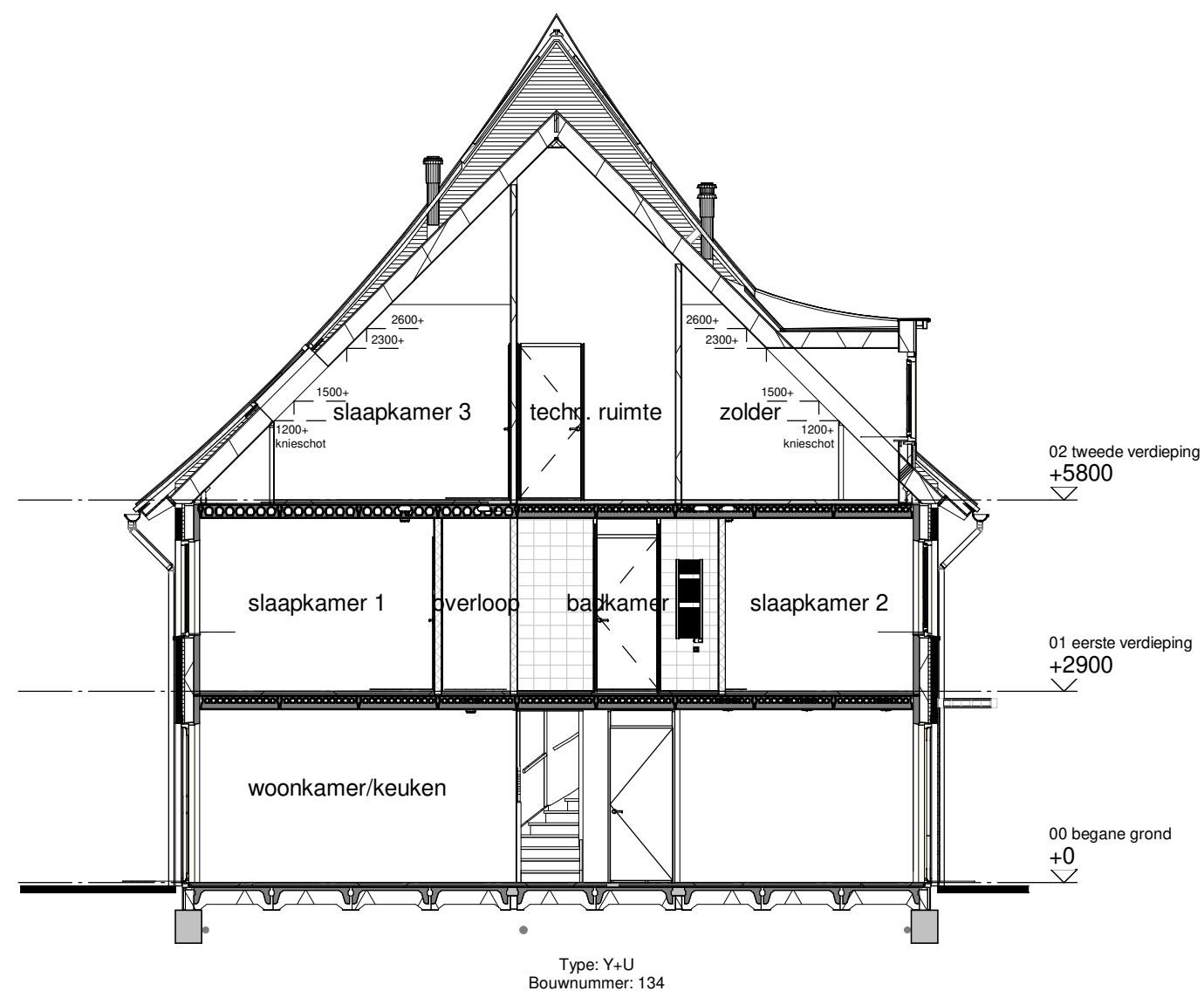
Doorsnede A
