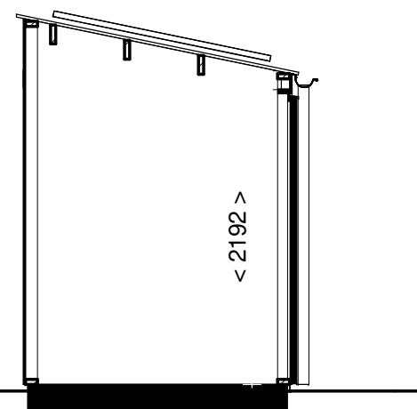
Doorsnede B-B
