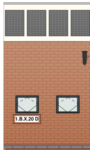
Vorgevel schaal 1:100
