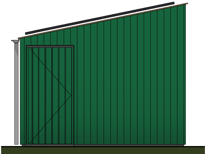
Rechter zijgevel
