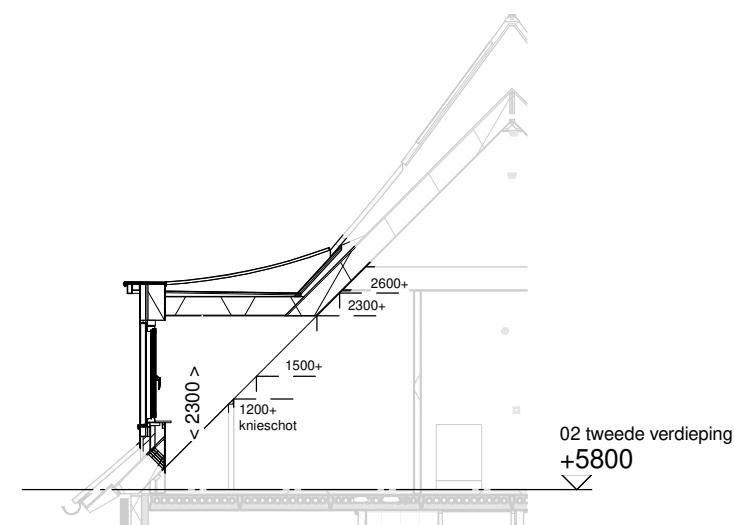
Doorsnede schaal 1:100
