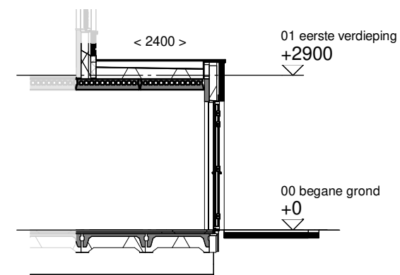
Doorsnede schaal 1:100
