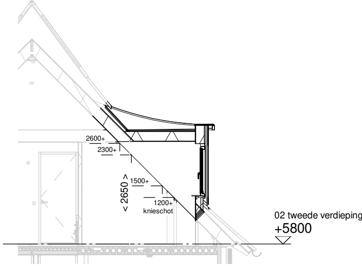
Doorsnede schaal 1:100
