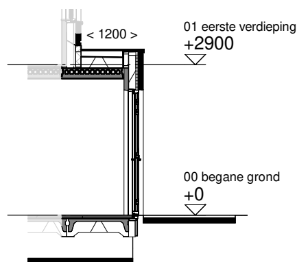
Doorsnede schaal 1:100
