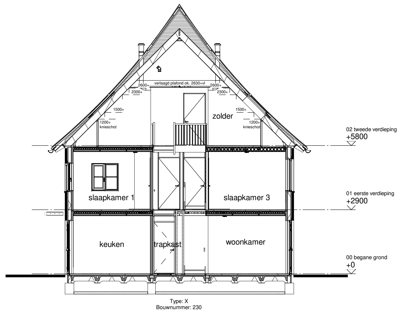
Doorsnede B
