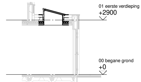
Doorsnede schaal 1:100
