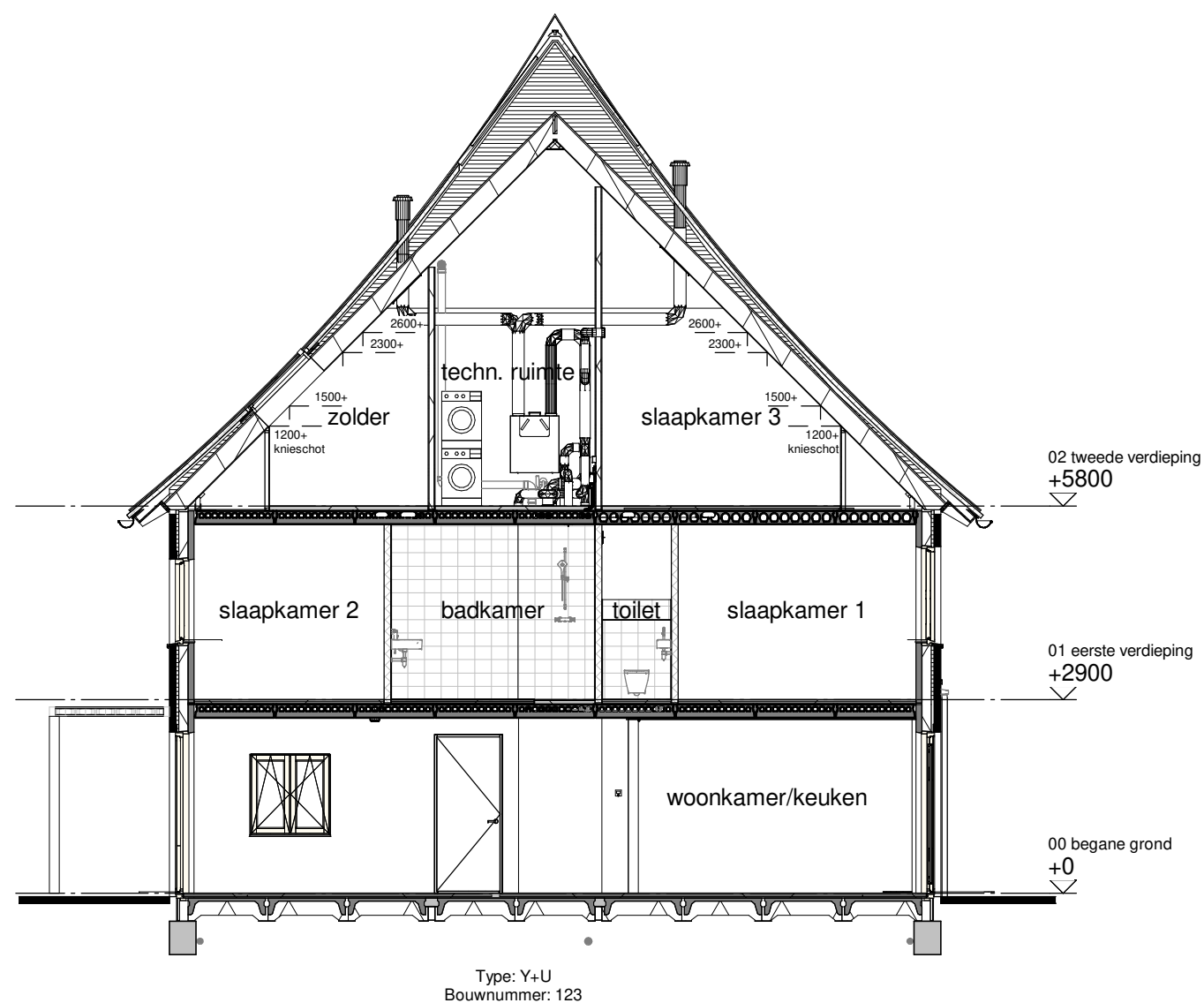
Doorsnede A
