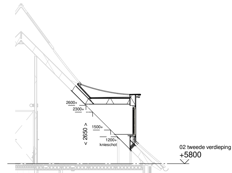
Doorsnede schaal 1:100
