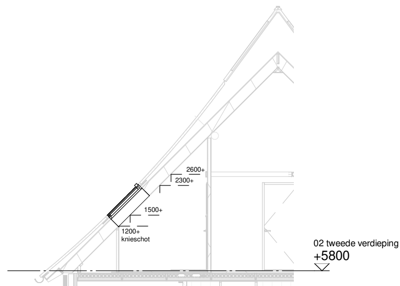
Doorsnede schaal 1:100
