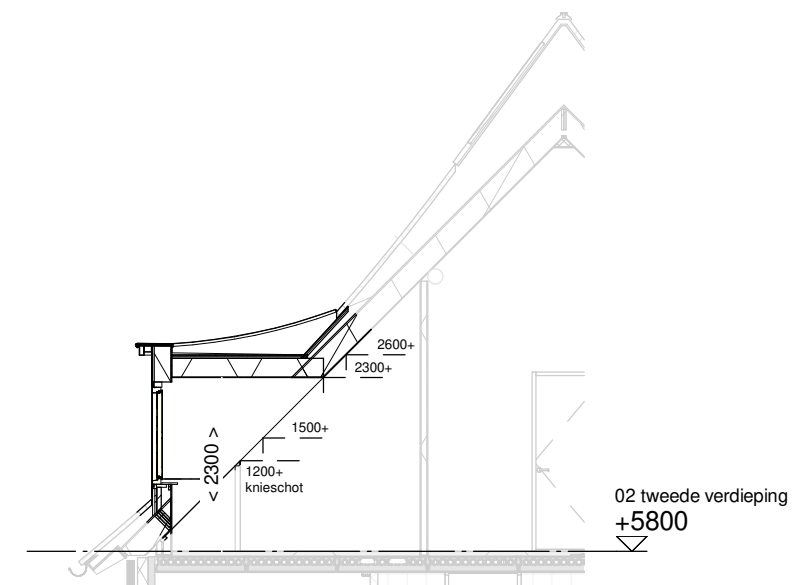
Doorsnede schaal 1:100
