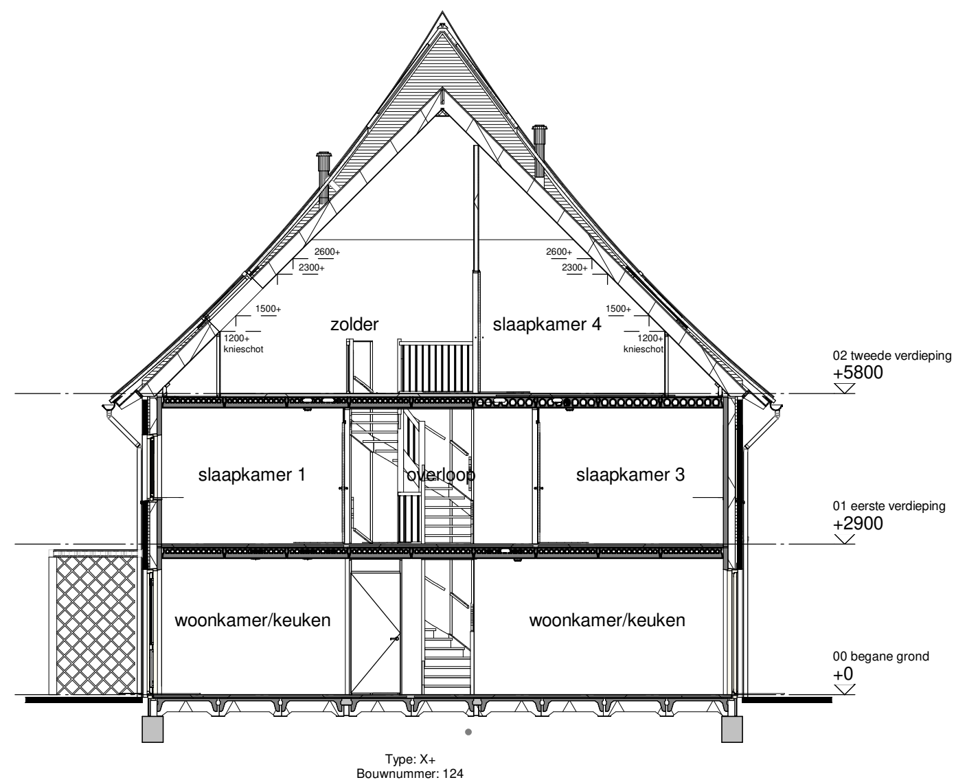
Doorsnede B
