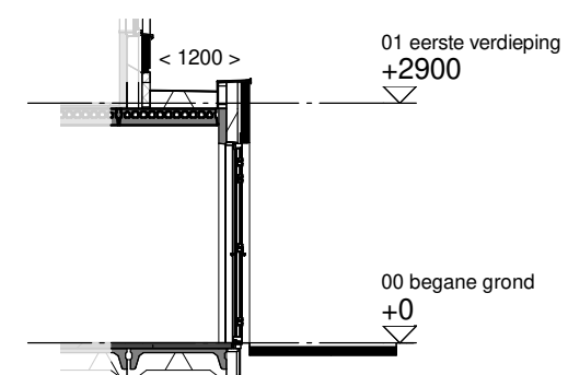
Doorsnede schaal 1:100
