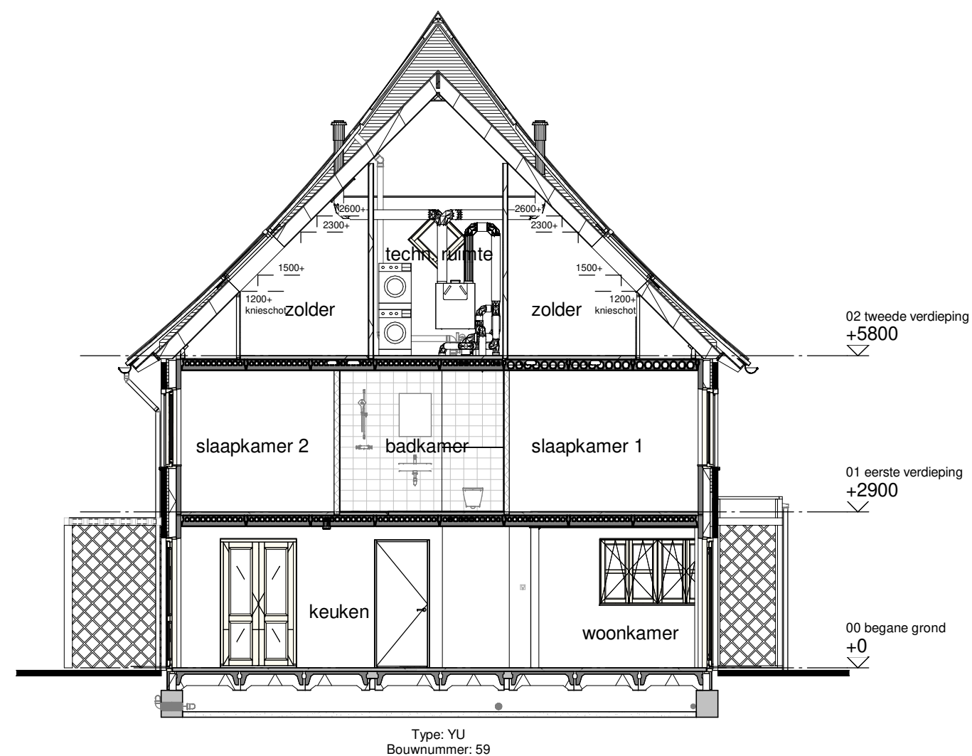
Doorsnede B
