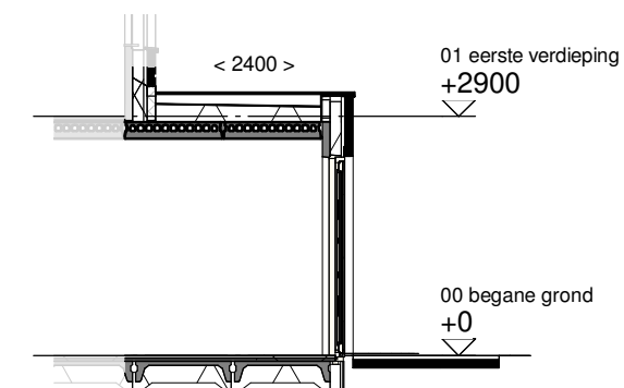
Doorsnede schaal 1:100
