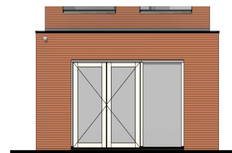
Achtergevel schaal 1:100
