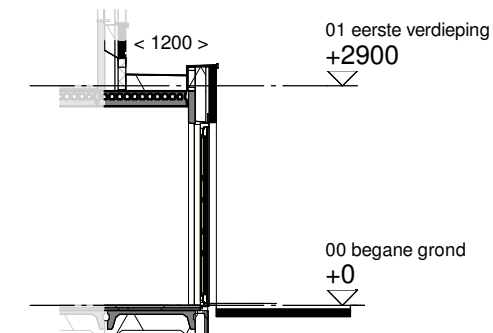
Doorsnede schaal 1:100
