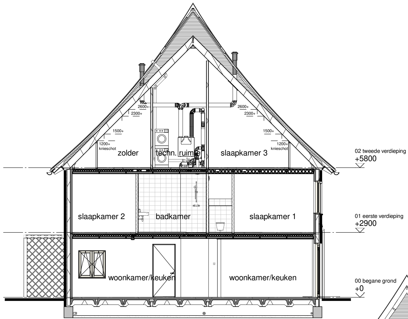
Doorsnede A
