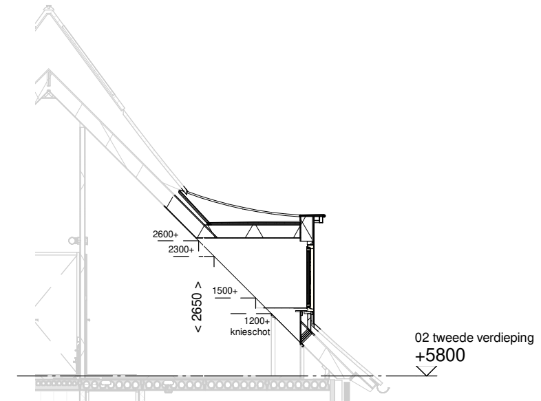
Doorsnede schaal 1:100
