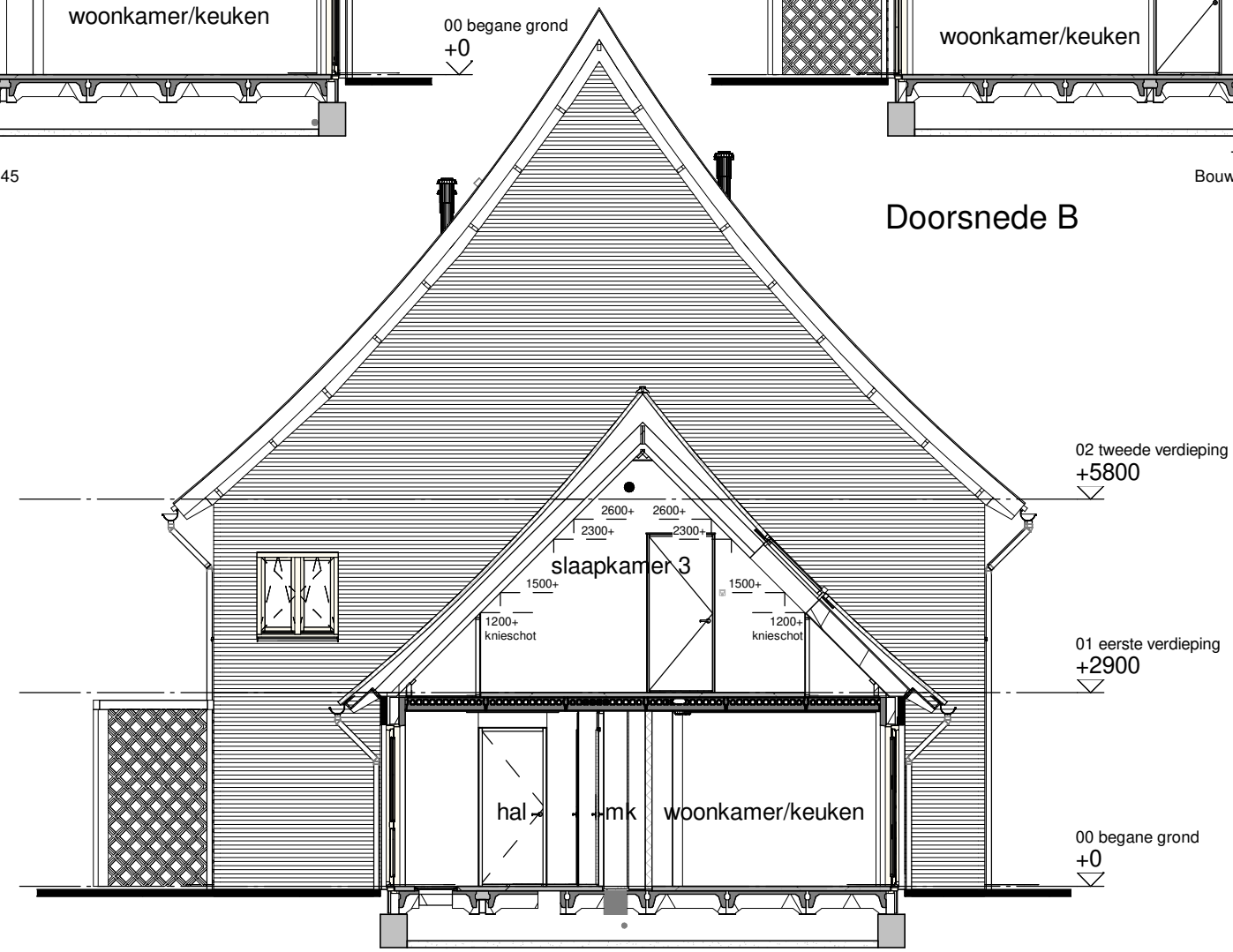
Doorsnede C
