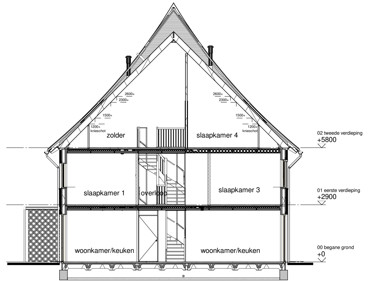
Doorsnede B
