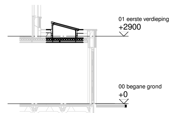
Doorsnede schaal 1:100
