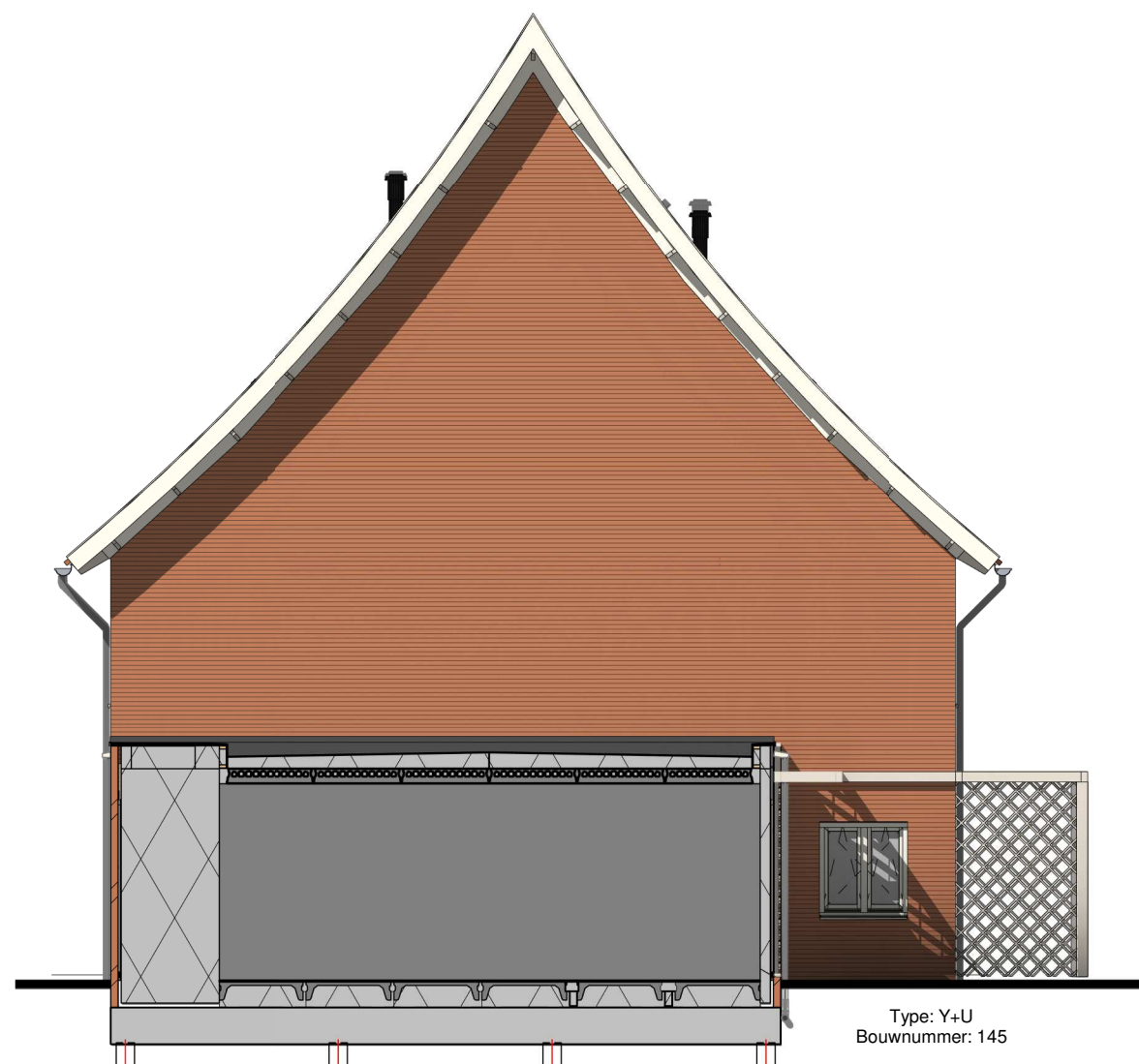
Linker zijgevel
