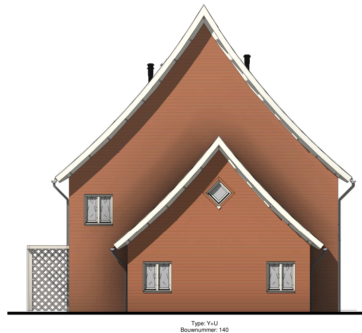
Rechter zijgevel
