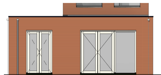
Achtergevel schaal 1:100
