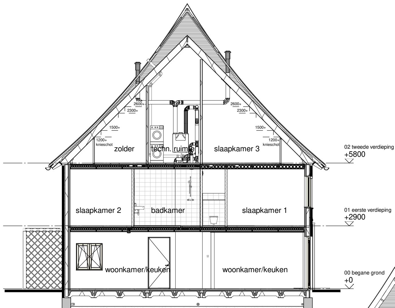
Doorsnede A
