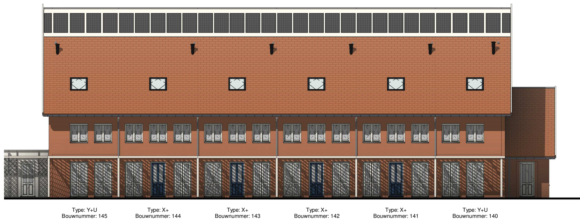
Voorgevel
