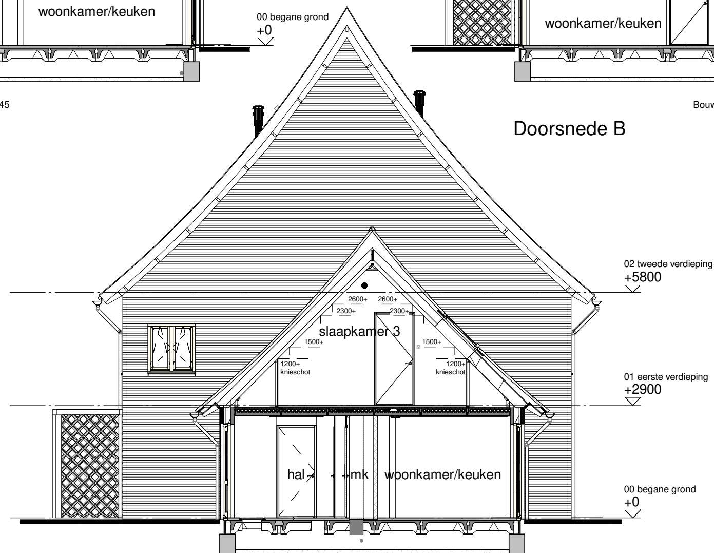
Doorsnede C
