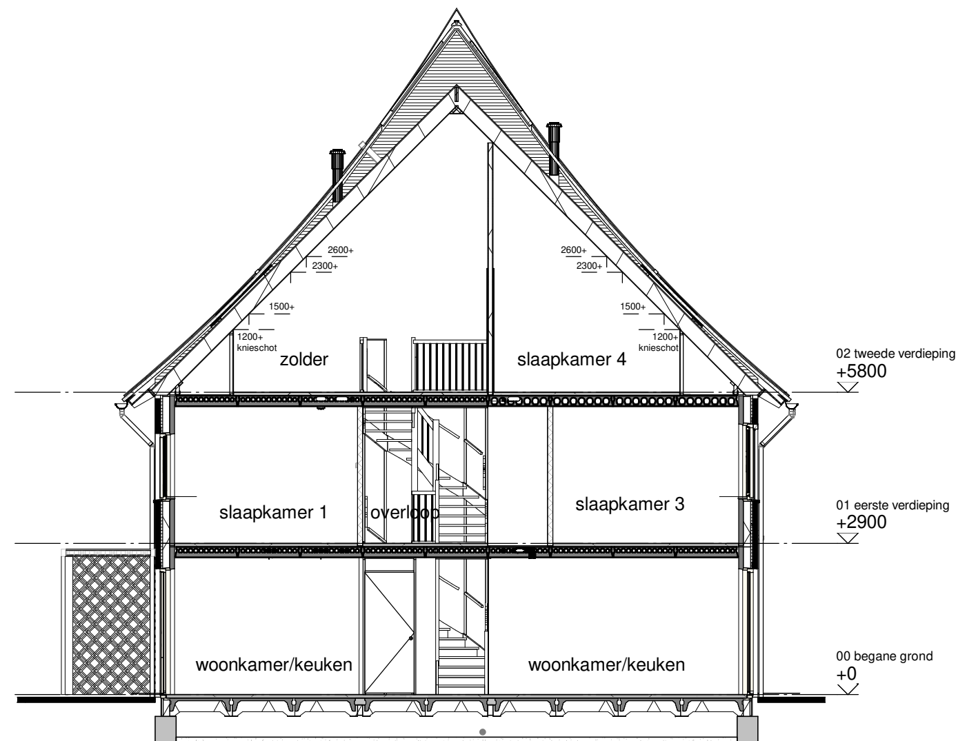
Doorsnede B
