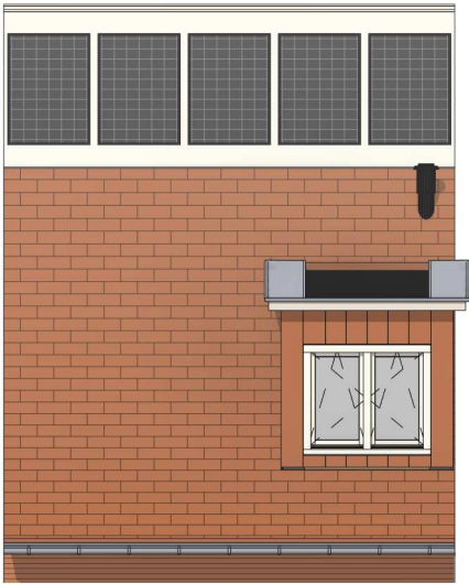
Achtergevel schaal 1:100
