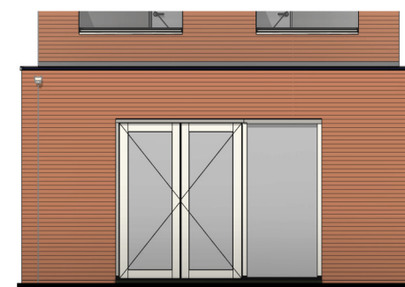
Achtergevel schaal 1:100
