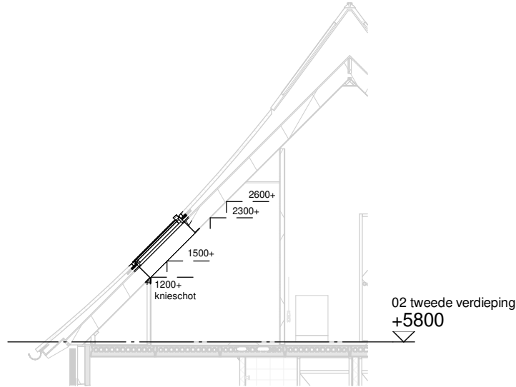
Doorsnede schaal 1:100
