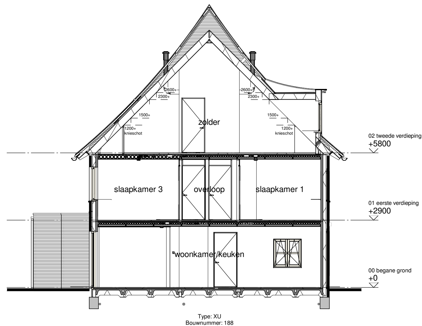
Doorsnede B
