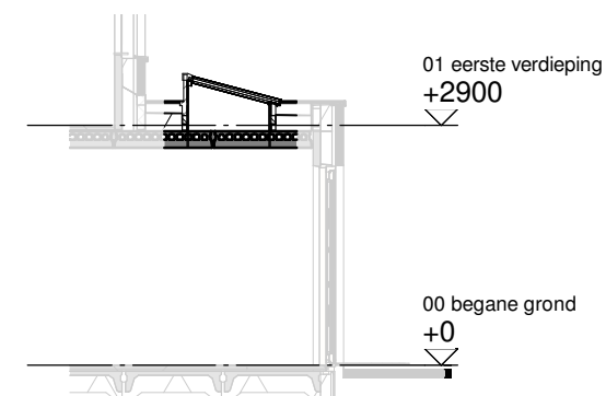
Doorsnede schaal 1:100
