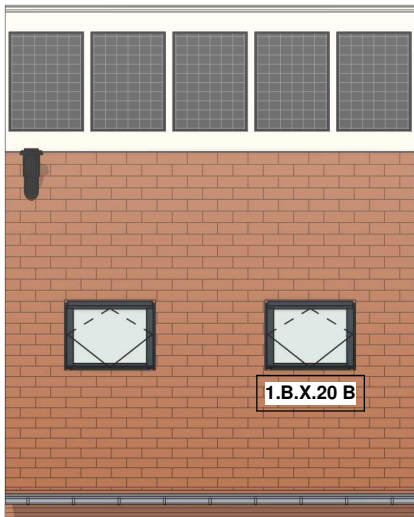
Achtergevel schaal 1:100
