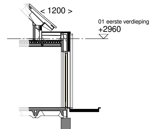
Doorsnede schaal 1:100
