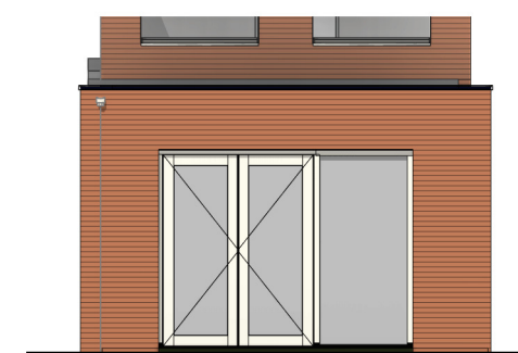
Achtergevel schaal 1:100
