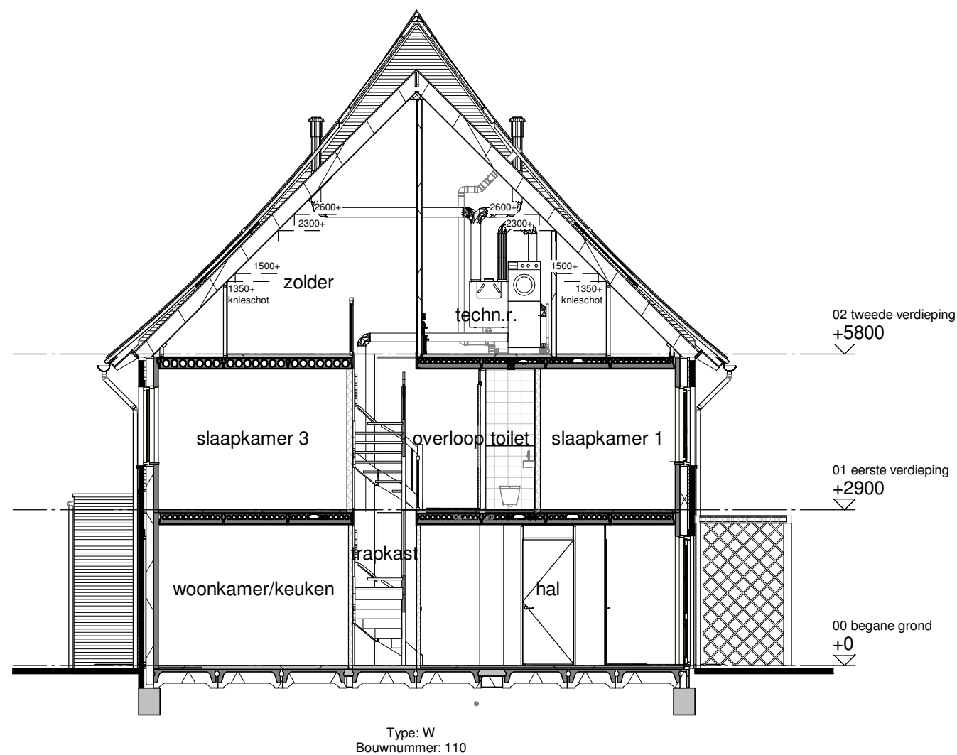
Doorsnede A
