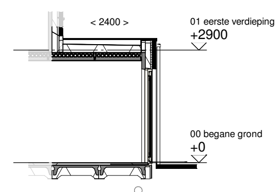
Doorsnede schaal 1:100
