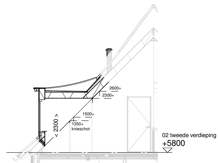
Doorsnede schaal 1:100
