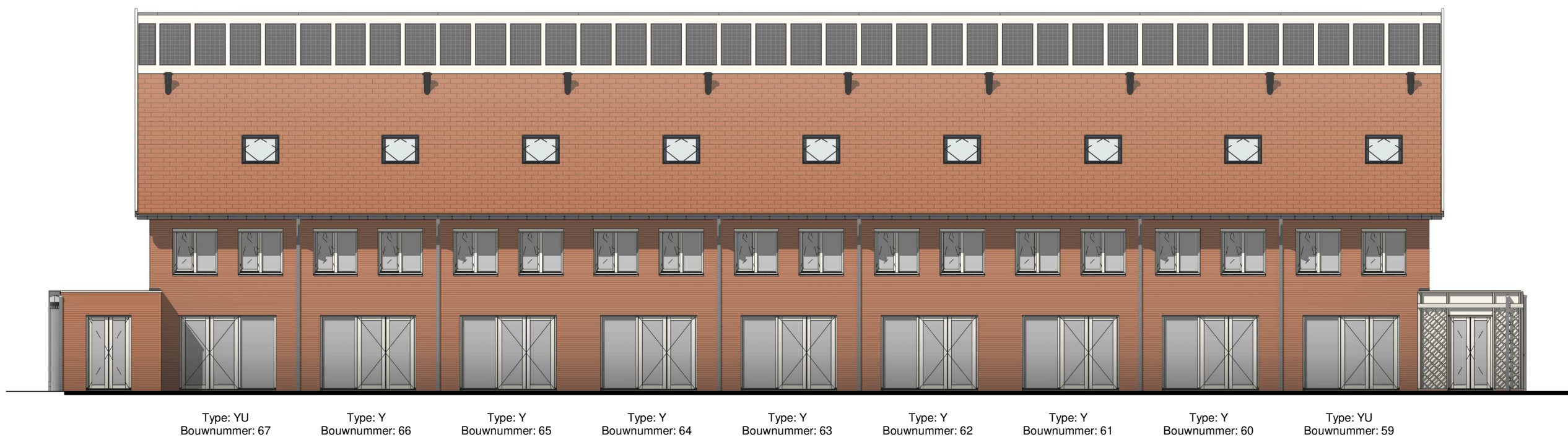
Achtergevel
