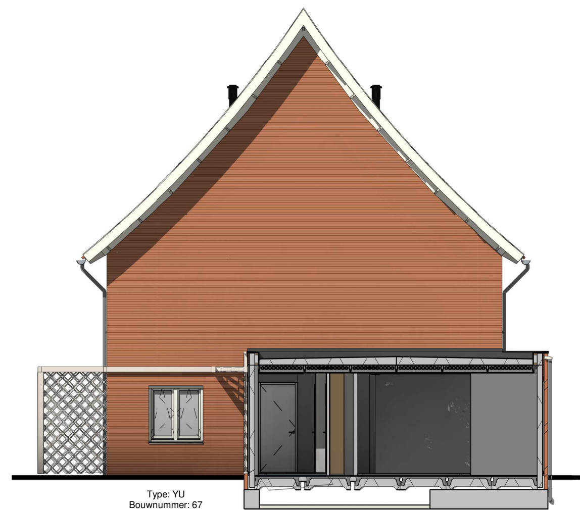
Rechter zijgevel
