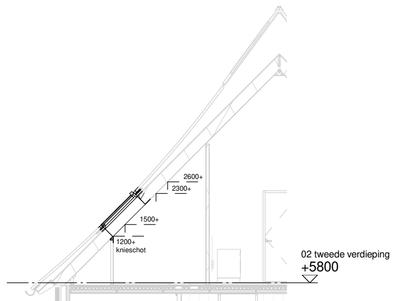
Doorsnede schaal 1:100
