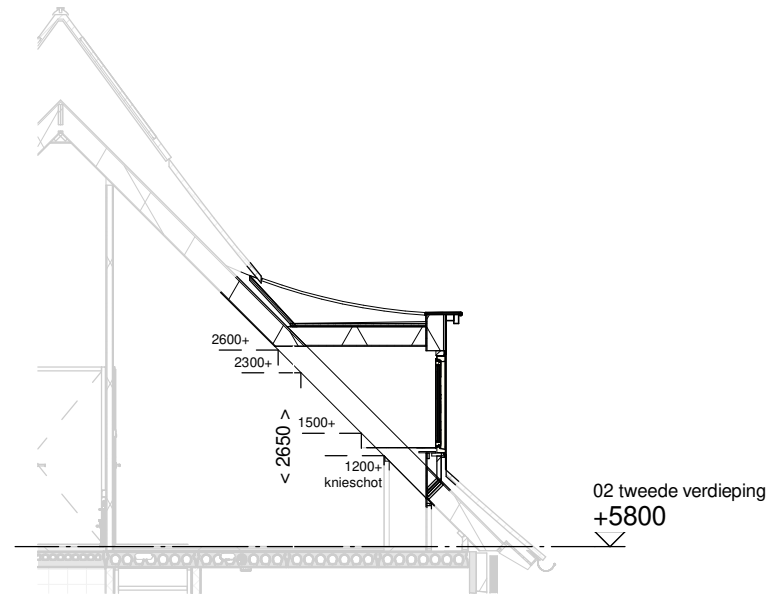
Doorsnede schaal 1:100
