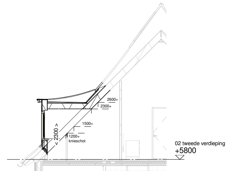
Doorsnede schaal 1:100
