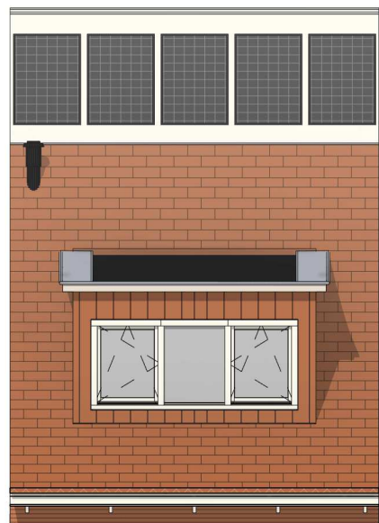
Achtergevel schaal 1:100
