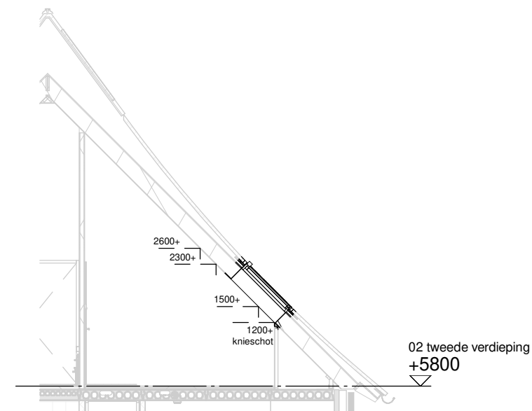
Doorsnede schaal 1:100
