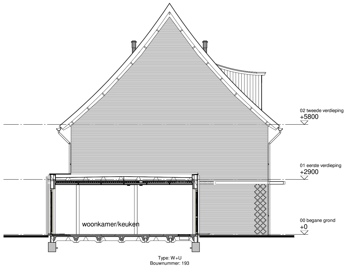
Doorsnede A
