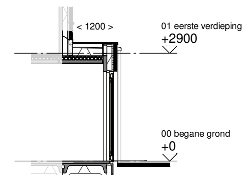
Doorsnede schaal 1:100
