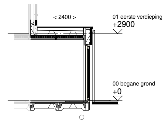
Doorsnede schaal 1:100
