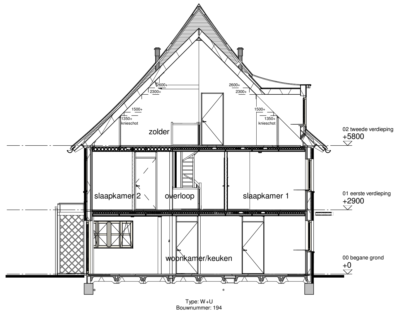
Doorsnede B
