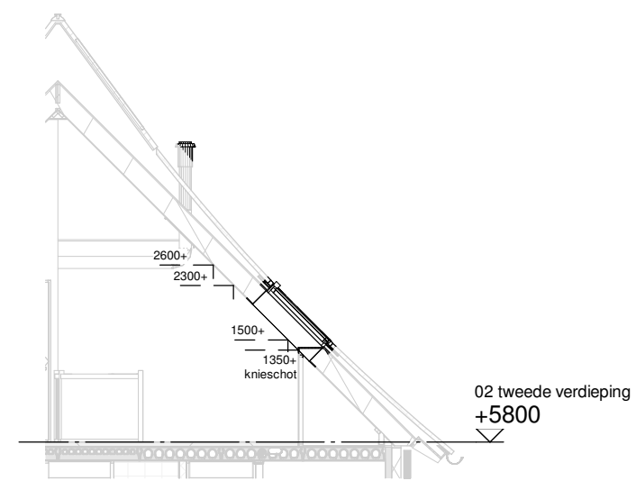
Doorsnede schaal 1:100
