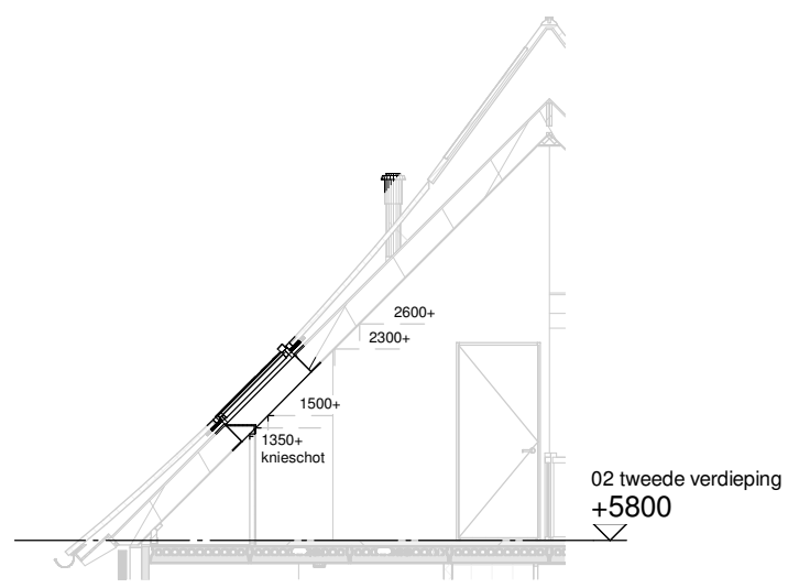
Doorsnede schaal 1:100
