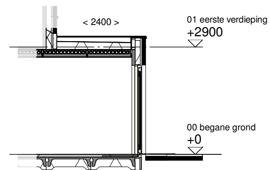
Doorsnede schaal 1:100
