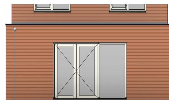
Achtergevel schaal 1:100
