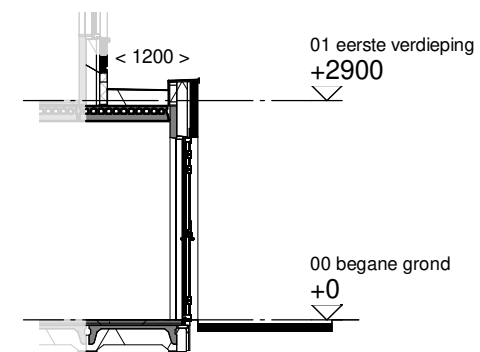
Doorsnede schaal 1:100
