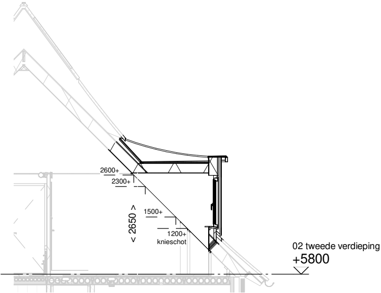
Doorsnede schaal 1:100
