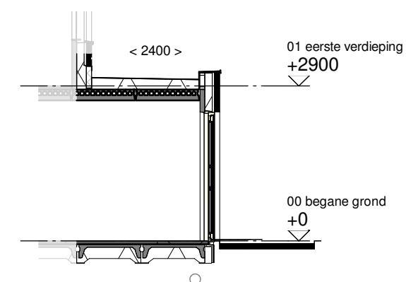
Doorsnede schaal 1:100
