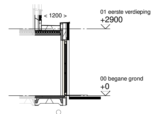
Doorsnede schaal 1:100
