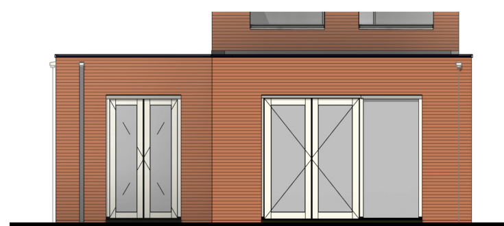
Achtergevel schaal 1:100
