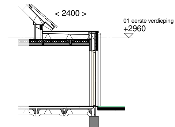
Doorsnede schaal 1:100
