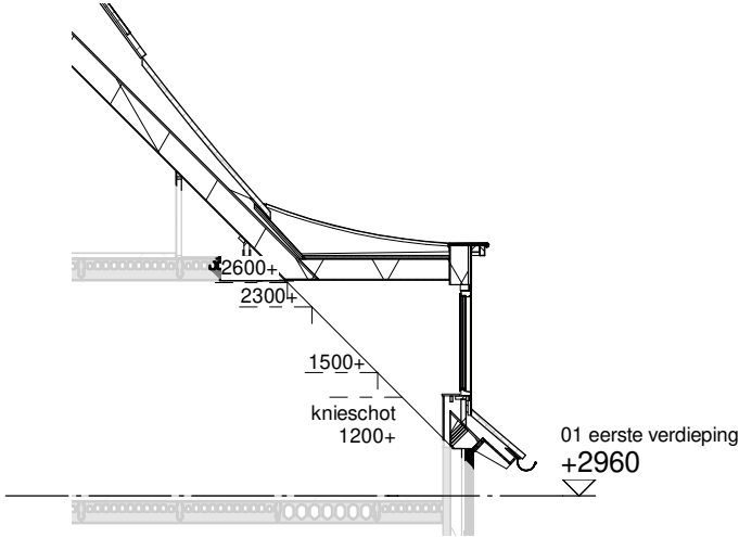
Doorsnede schaal 1:100
