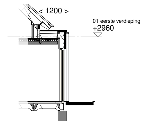
Doorsnede schaal 1:100
