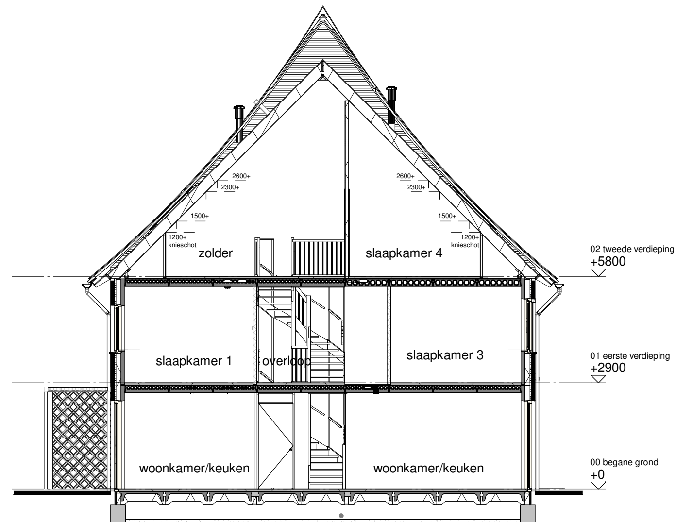
Doorsnede B
