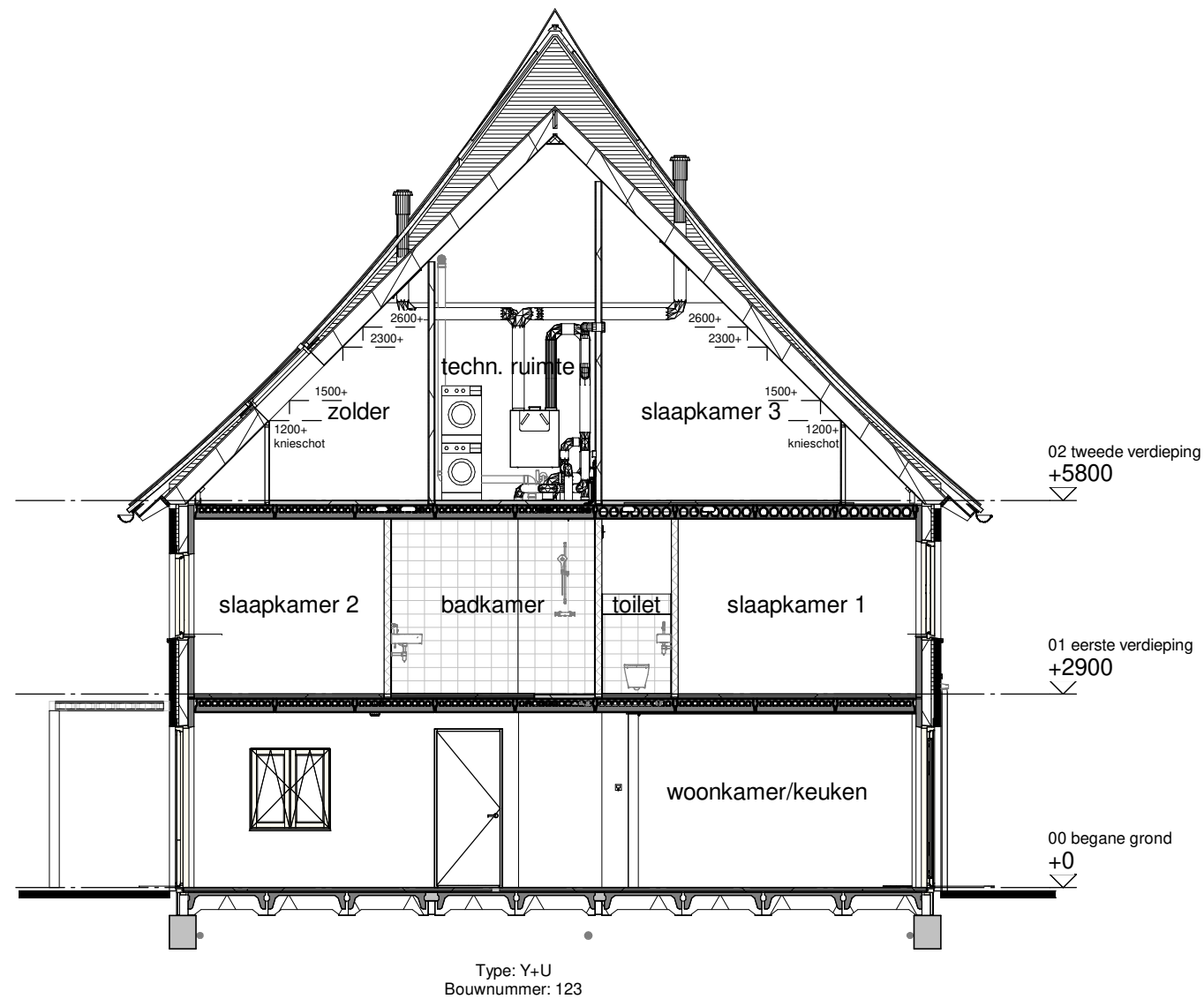
Doorsnede A
