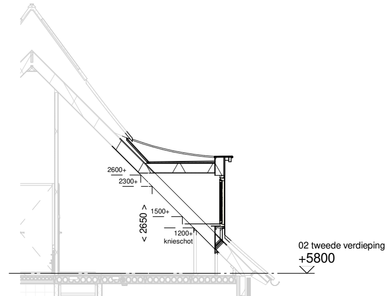
Doorsnede schaal 1:100
