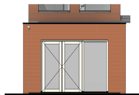
Achtergevel schaal 1:100
