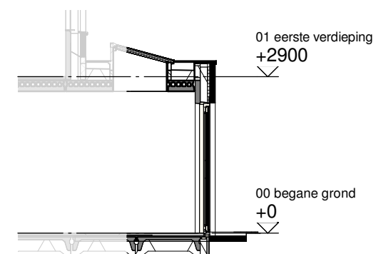
Doorsnede schaal 1:100
