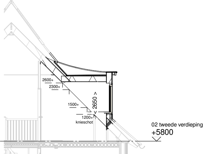
Doorsnede schaal 1:100
