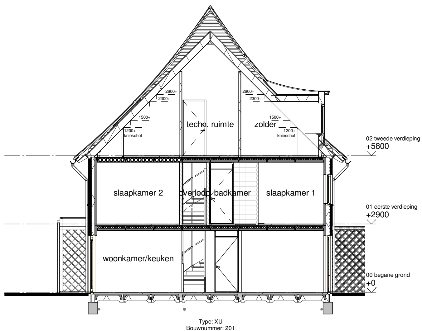
Doorsnede A
