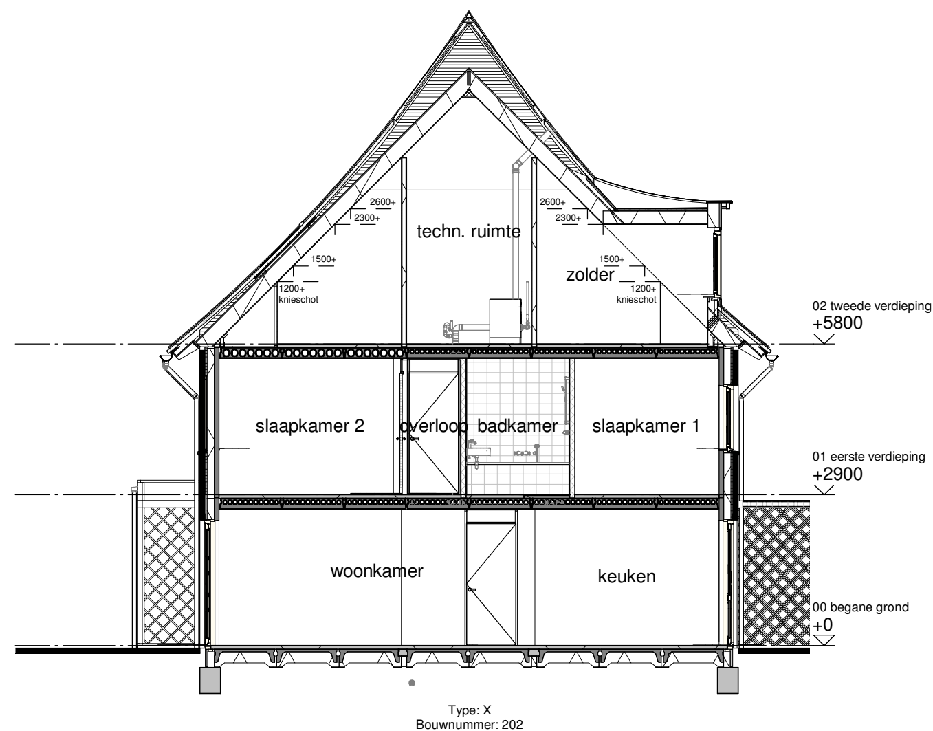
Doorsnede B
