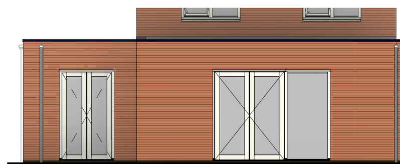
Achtergevel schaal 1:100
