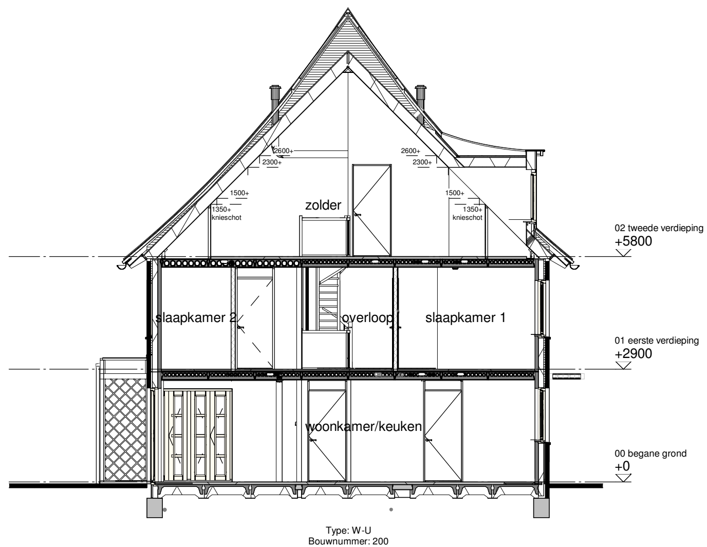
Doorsnede A
