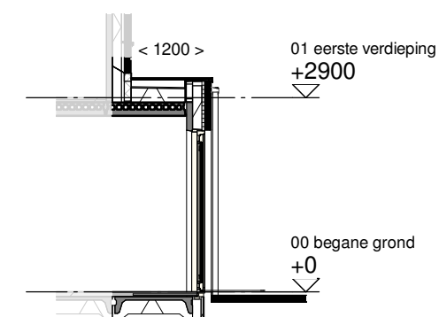
Doorsnede schaal 1:100
