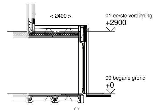
Doorsnede schaal 1:100
