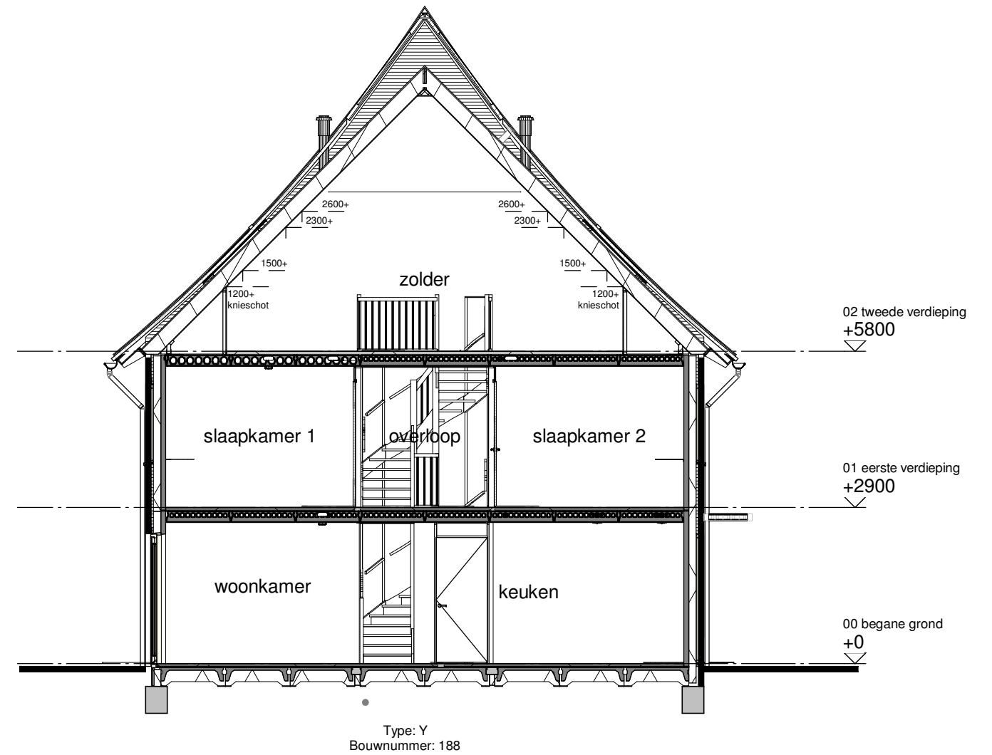
Doorsnede B
