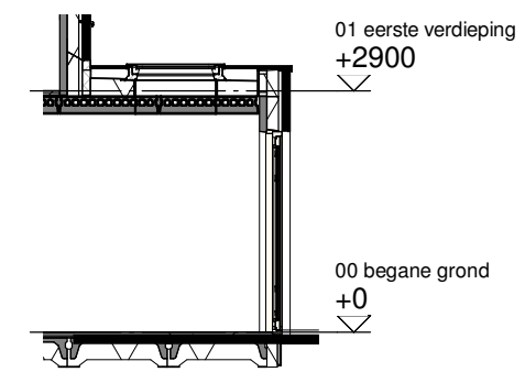
Doorsnede schaal 1:100
