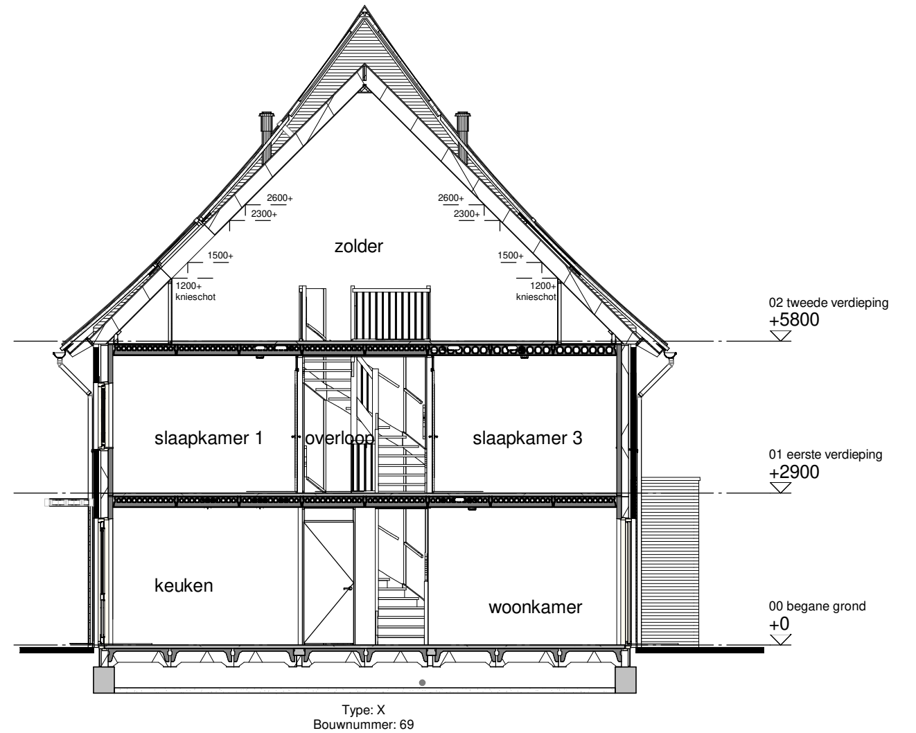
Doorsnede B
