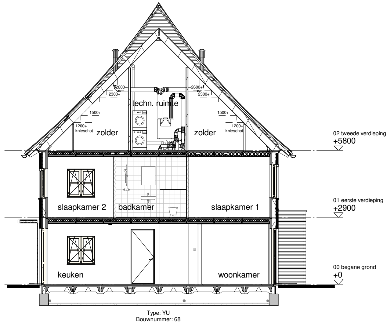
Doorsnede A
