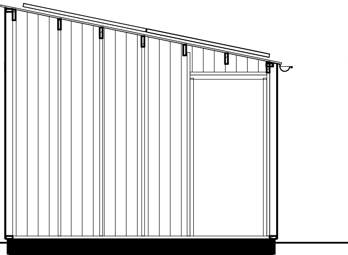
Doorsnede B-B
