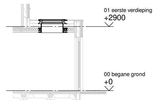
Doorsnede schaal 1:100
