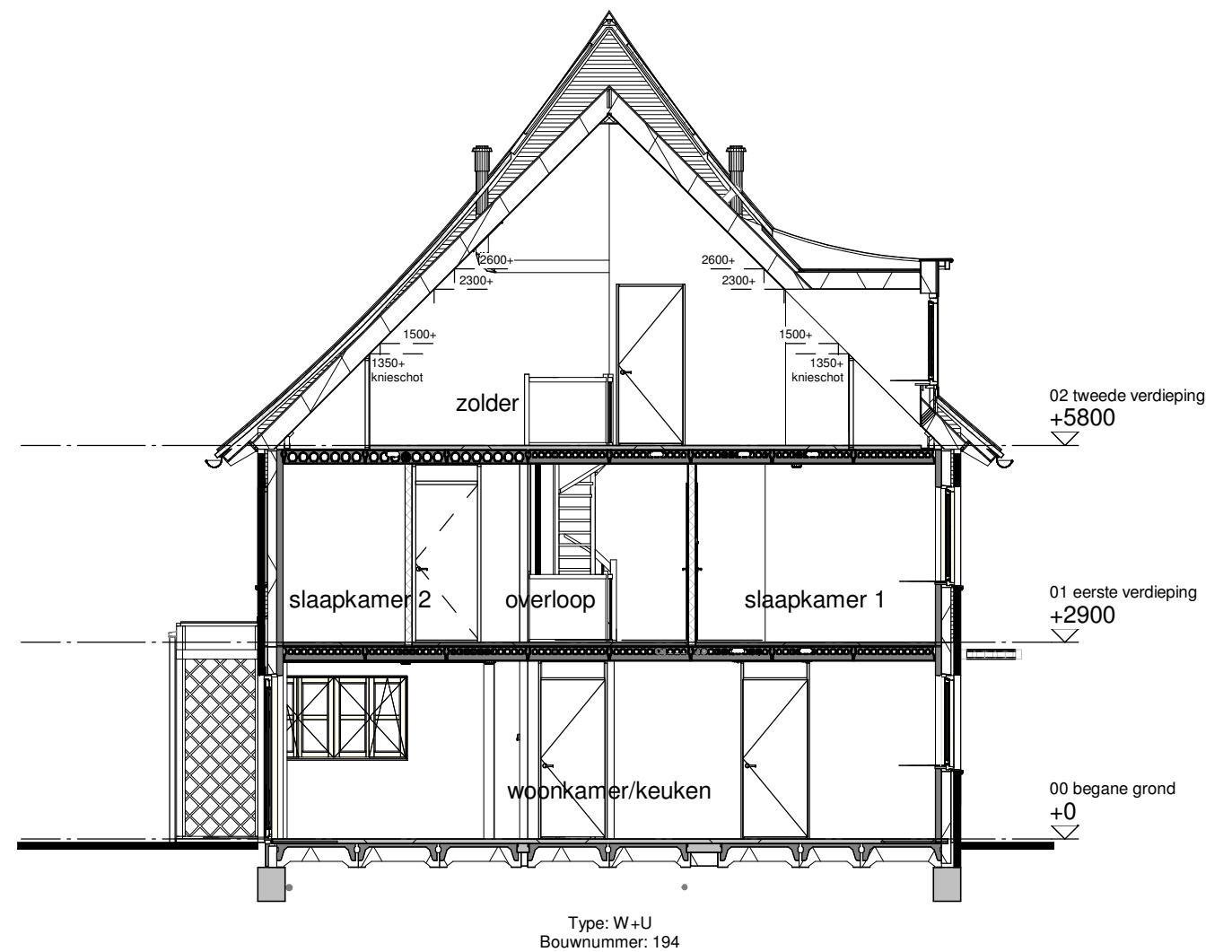
Doorsnede B
