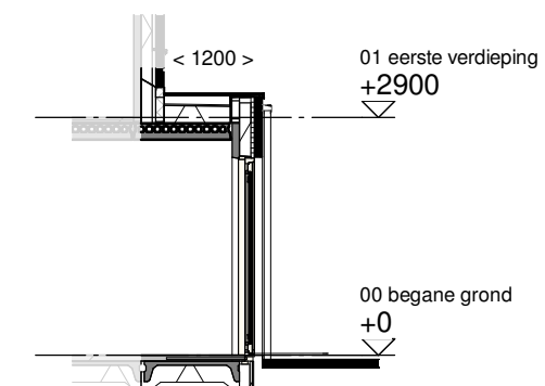
Doorsnede schaal 1:100
