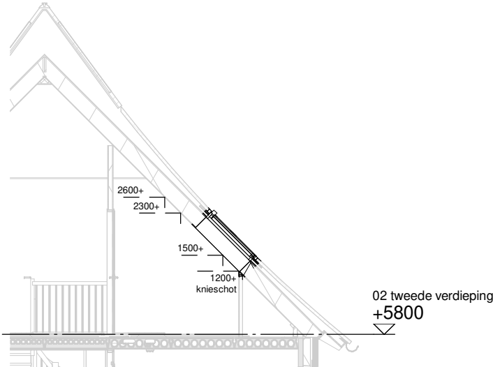
Doorsnede schaal 1:100
