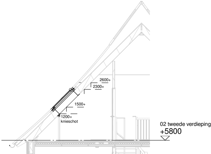
Doorsnede schaal 1:100
