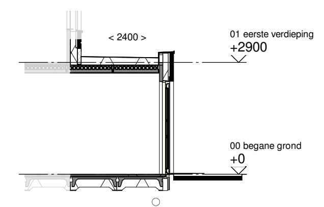
Doorsnede schaal 1:100
