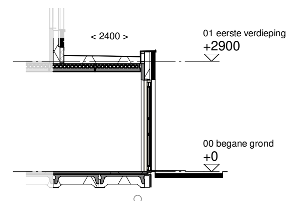
Doorsnede schaal 1:100
