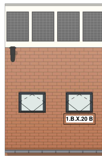
Achtergevel schaal 1:100
