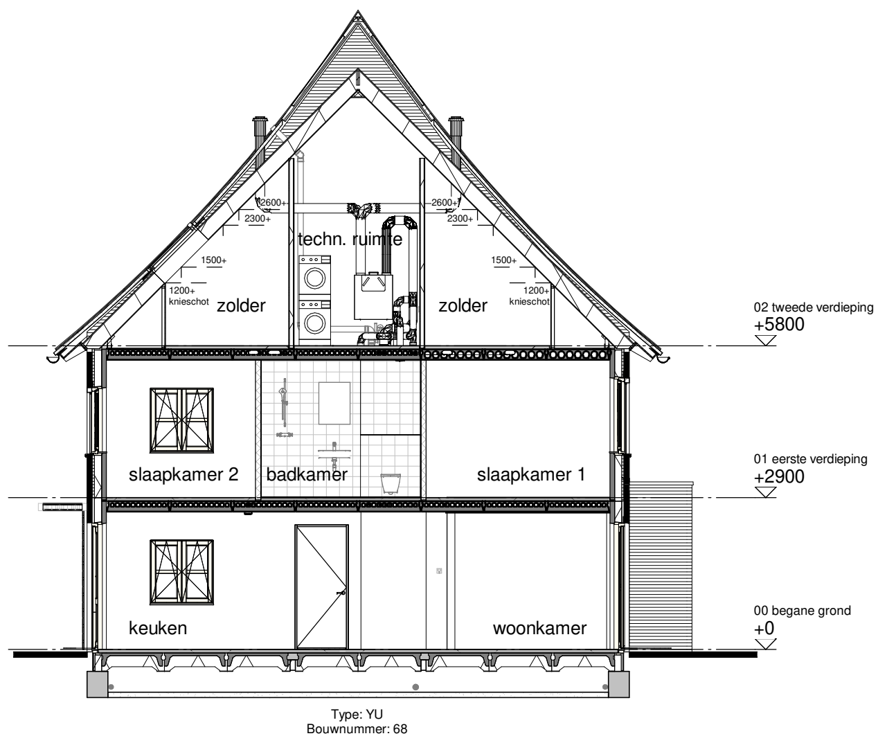
Doorsnede A
