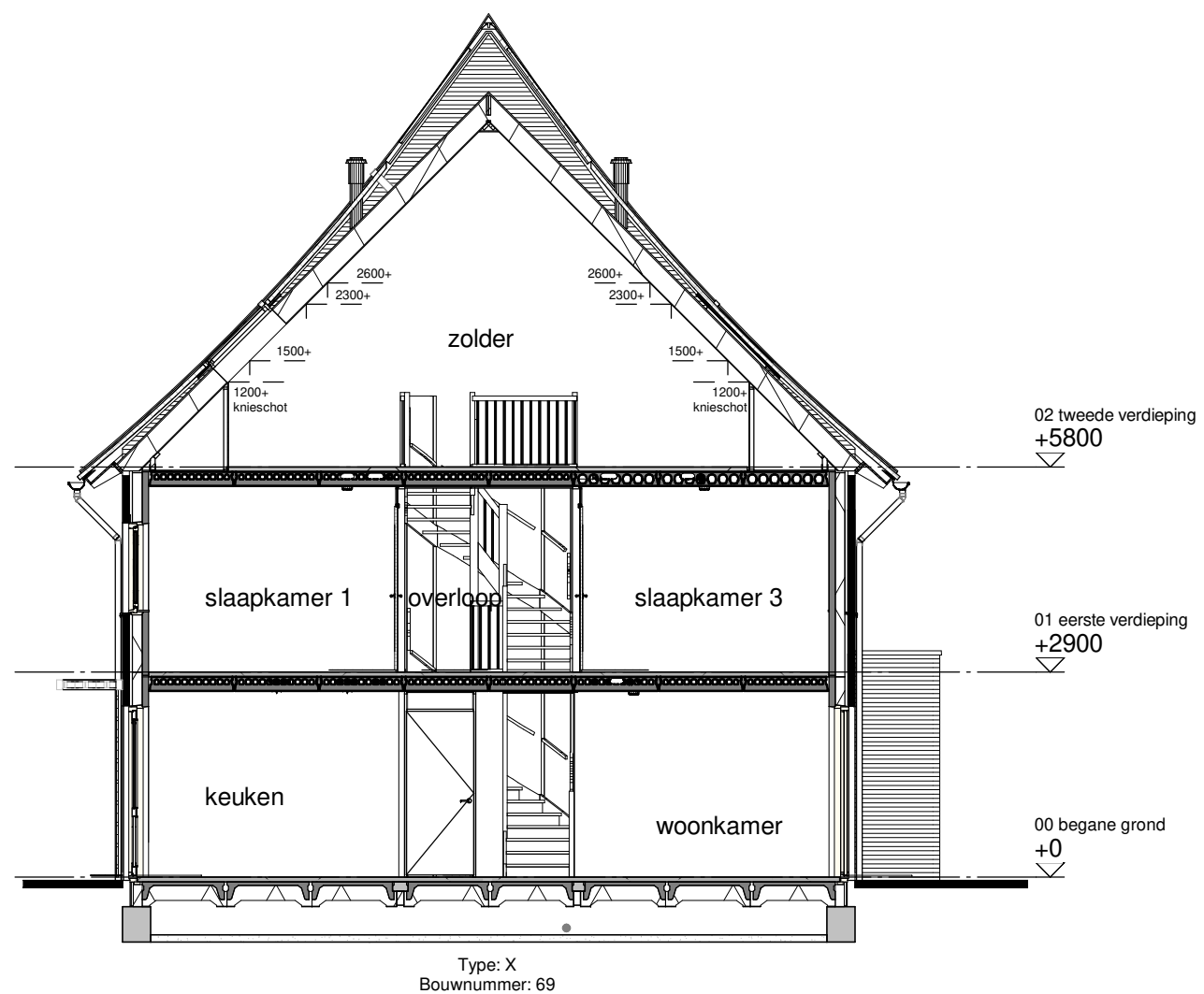
Doorsnede B
